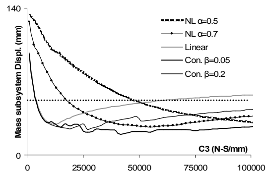
شکل ۱۰: حداکثر تغییر مکان زیر سازه جرمی در زلزله السترو.
