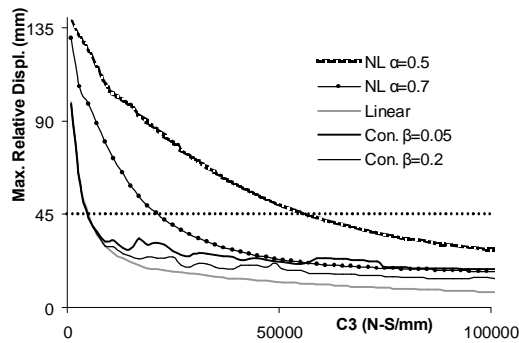
شکل ۱۱: حداکثر تغییر مکان نسبی دو زیرسازه در زلزله السترو.
