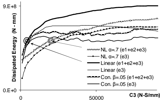
شکل ۱۴: اتلاف انرژی در سازه (e1+e2) و در میراگرمیانی e3 در زلزله الستترو.
