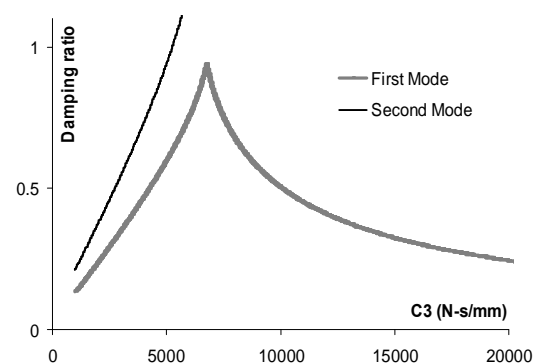
شکل ۷: نمودار تغییرات نسبت میرایی بر حسب C_3 .
