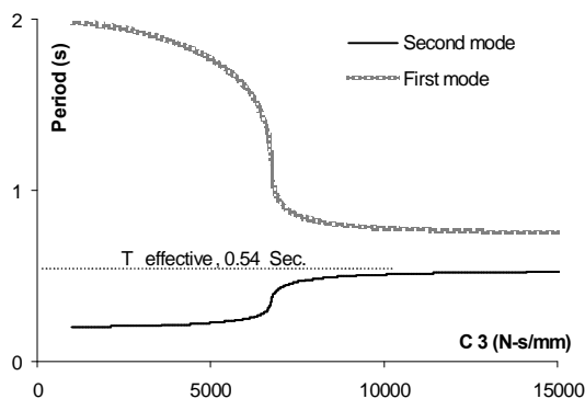
شکل ۸: تغییرات پریود دومود سازه بر حسب C_3 .
