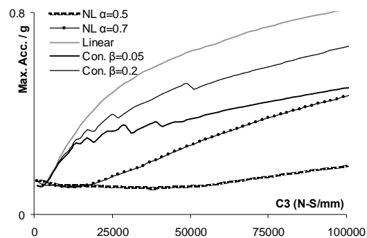
شکل ۱۶: حداکثر شتاب سازه نرم در زلزله الاستترو.
