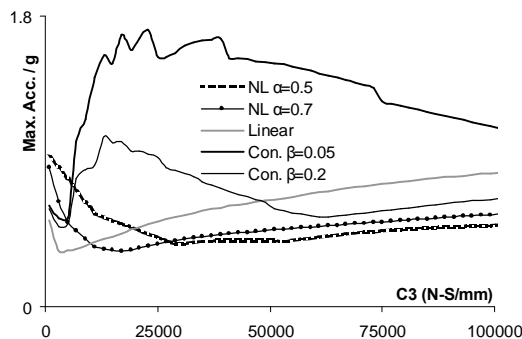
شکل ۱۵: حداکثر شتاب سازه سخت در زلزله الستترو.
