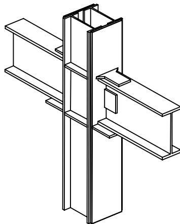
شکل ۱: نمای سه بعدی ستون های مرکب مزدوج I شکل به- همراه اتصالات گیردار.
