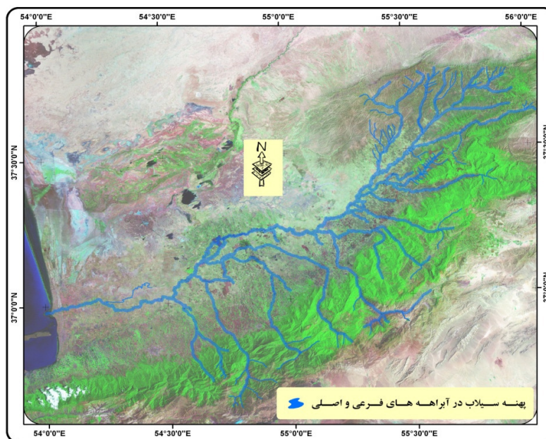
شکل ۸) پهنه‌های در معرض آب‌گرفتگی ناشی از سیلاب
