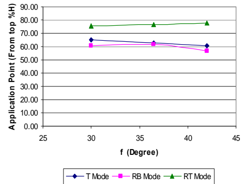
شکل ۱۴: تأثیر زاویه اصطکاک داخلی خاک بر نقطه اثر برآیند توزیع فشار مقاوم در اعماق مختلف.
