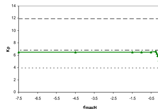
شکل ۶: تغییرات ضریب رانش افقی خاک.
