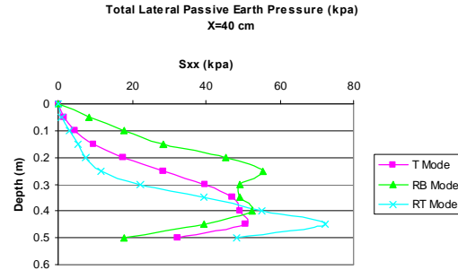
شکل ۲۲: تأثیر نوع تغییر مکان دیوار بر توزیع فشار مقاوم خاک بر دیوار در اعماق مختلف.
