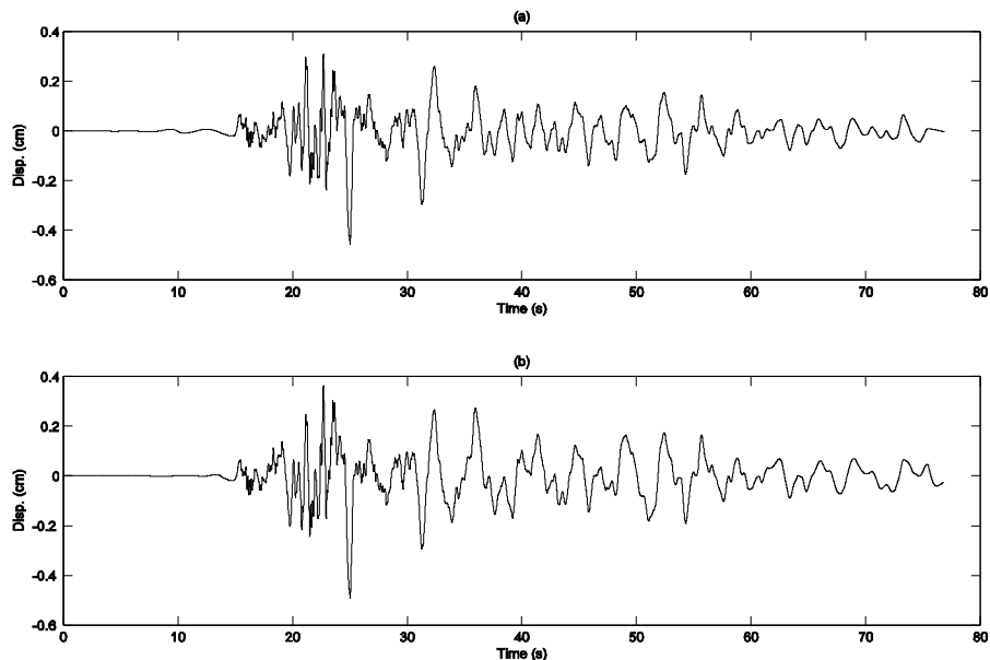
شکل ۸: سیگنال جابجایی Comp T از زلزله سیلاخور که در ایستگاه دره اسپار ثبت شده است. (a) تصحیح شده توسط روش مرسوم و با تصحیح خط پایه (پیش حادثه نامناسب و بیشینه آن: -0.457). (b) تصحیح شده توسط موجک و بدون تصحیح خط پایه (پیش - حادثه مناسب و بیشینه آن: -0.492).
