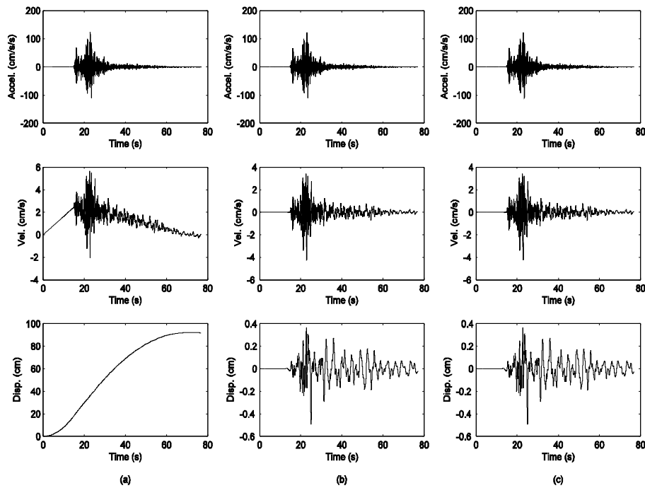
شکل ۷: Comp T از زلزله سیلاخور که در ایستگاه دره اسپار ثبت شده است. (a) سیگنال اصلی ثبت شده. (d) سیگنال تصحیح شده توسط تبدیل موجک بدون تصحیح خط پایه (خوب). (e) سیگنال تصحیح شده توسط تبدیل موجک بعد از تصحیح خط پایه (خوب). (اعمال Sym8 مرتبه ۸ بر سیگنال شتاب و Sym8 مرتبه ۹ بر سیگنال سرعت).
