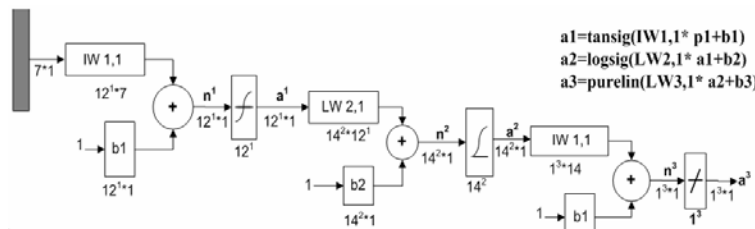
نمودار ۳. پیکره بندی شبکه مدل عصبی فرآیند اسپری درآیننگ
