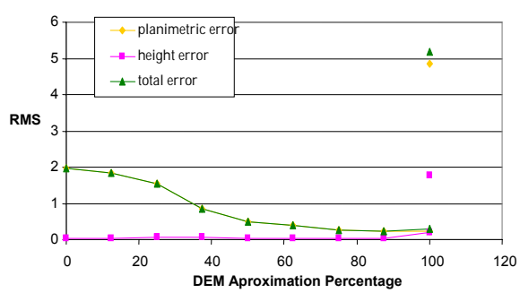
شکل ۱۱: نمودار انحراف معیار خطاهای نقاط چک در DEM با دامنه اختلاف ارتفاع ۴۰۰ متر (واحد بر حسب متر).
