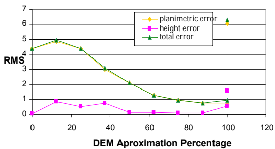
شکل ۱۰: نمودار انحراف معیار خطاهای نقاط چک در DEM با شیب بیشینه ۲۷٪ (بر حسب متر).
