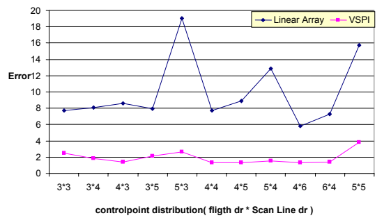
شکل ۱۳: نمودار انحراف معیار خطاها در تصویر آرایه خطی و تصویر VSPI در حالت‌های مختلف توزیع نقاط کنترل.
