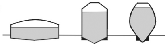
تصویر ۸- یکپارچگی سازه و عملکرد در مخازن. ماخذ: (Prestressed concrete design and construction 2nd edn. Wilhelm Ernst, Berlin, 546)
