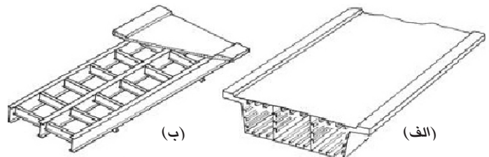
تصویر ۹- پیشرفت یکپارچگی فرم و عملکرد سازه‌ای: (الف) ساخت پل قدیمی که در آن سطح پل به طور مجزا روی تیرها و تیرهای متقاطع بین روی تیرهای اصلی قرار می‌گیرند، (ب) ساخت امروزی پل که در آن سطح پل نه تنها نیروهای را پخش می‌کند، بلکه به عنوان جان فوقانی تیر با مقطع قوطی نیز عمل می‌کند. ماخذ: (Art of Structural Design, Holgate, A. 1986)
