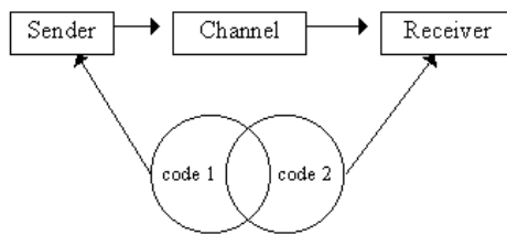
(۲) الگوی مولز
