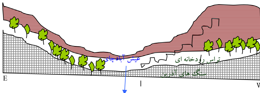
شکل ۳- مقطعی از موقعیت زمین شناسی و ژئومورفولوژیکی روستای عیش آباد
