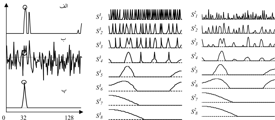
شکل ۹: توابع S_j^2 محاسبه شده برای سیگنال نویزی شکل ۷ (ب).
