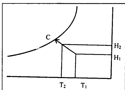
تصویر شماره ۱. روند خنک‌سازی از طریق تبخیر در جدول سایکرومتریک
