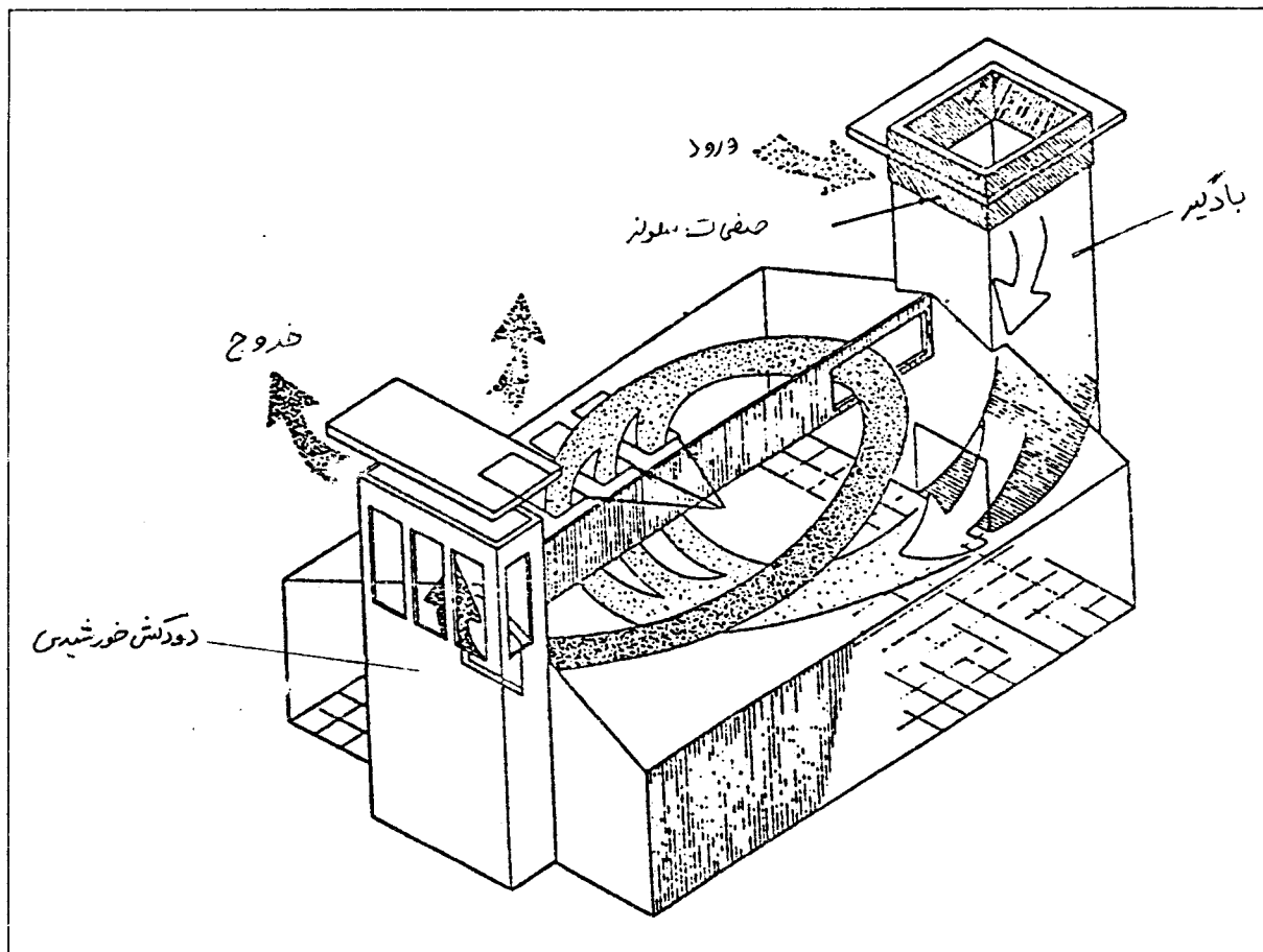
تصویر شماره ۴. سیستم ورود هوای مرطوب از طریق بادگیر و خروج از طریق دودکش خورشیدی (۳)
