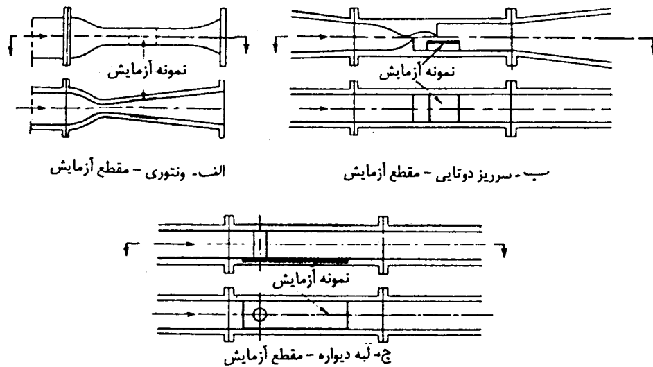
شکل ۵: انواع مختلف محفظه‌های کاری مورد استفاده در لوله‌های متقارب.
