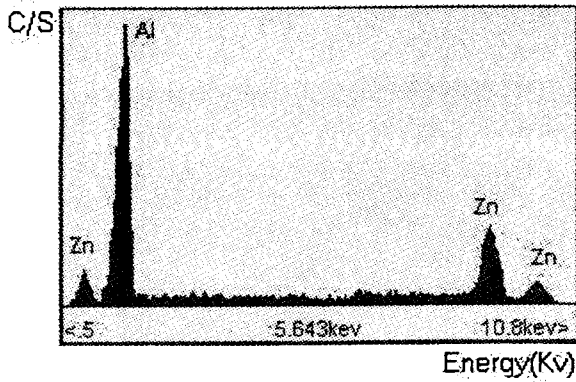
شکل ۲۰: طیف میکروسکوپی (E.D.A) از فاز زمینه شکل ۱۰، میکروسکپ الکترونی (S.T.E.M).
