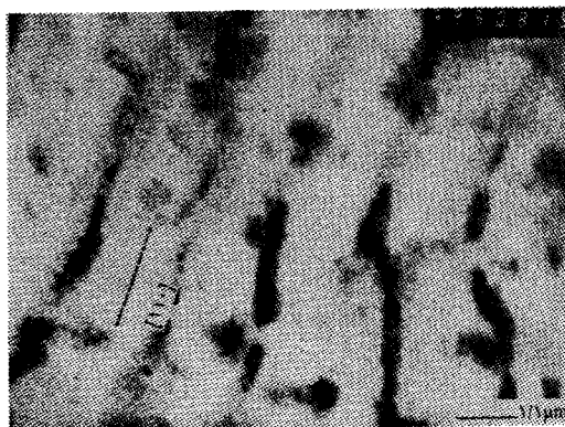
شکل ۴: ساختار میکروسکوپی از شمش پیرشده در دمای محیط به مدت سه ماه نشان دهنده رشد فاز های رسوبی به موازات جهت [۱۱۰]، در ساختاری با محور پراش <۱۱۲>. میدان روشن.
