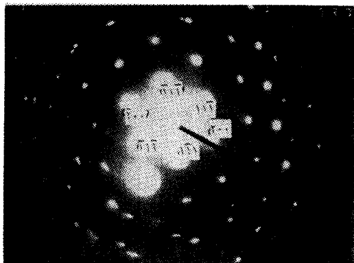
شکل ۹: الگوی پراش از شکل ۸، محور پراش \langle 110 \rangle .
