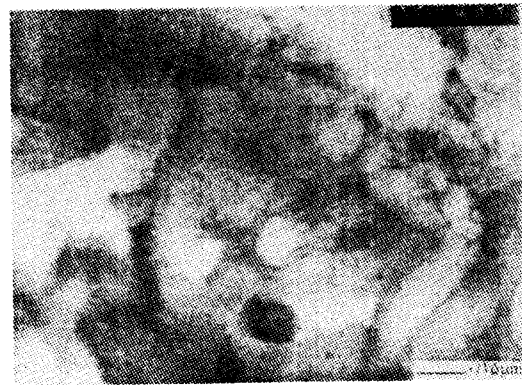
شکل ۱۷: ساختار میکروسکوپی از شمش پیرشده در دمای 100^{\circ}\text{C} به مدت ۱۴۴۰ دقیقه. نشان دهنده ذرات گلوله ای شکل، میدان روشن.
