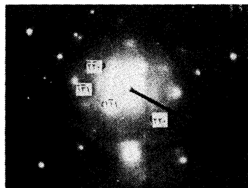
شکل ۱۲: الگوی پراش از شکل ۱۱، محور پراش <۱۱۲>.
