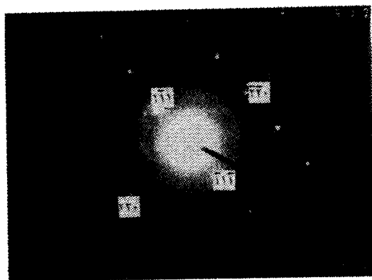
شکل ۵: الگوی پراش از شکل ۴، محور پراش <۱۱۲>.
