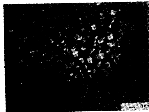
شکل ۳: ساختار میکروسکوپی از شکل ۱ میدان تاریک از نقطه (۲۲۰) از الگوی پراش شکل ۲.
