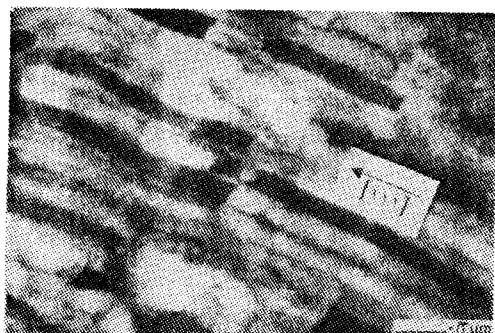
شکل ۱۰: ساختار میکروسکوپی از شمش پیرشده در دمای 100^\circ\text{C} به مدت ۱۴۴۰ دقیقه، نشان دهنده مجزا شدن رسوبات غنی از روی به صورت صفحه ای میدان روشن.
