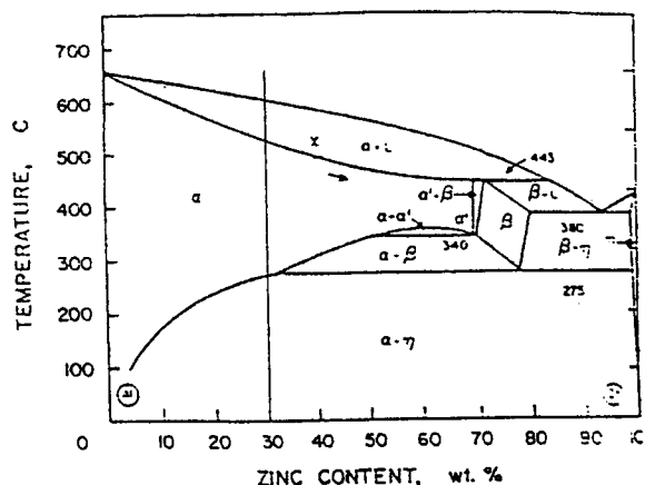
شکل ۲۲: نمودار فازی آلومینیم - روی .
