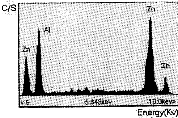
شکل ۲۱: طیف میکروسکوپی (E.D.A) از فاز رسوبی از شکل ۱۰، میکروسکپ الکترونی (S.T.E.M).
