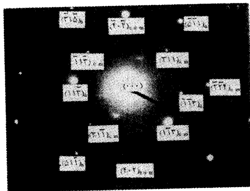
شکل ۱۸: الگوی پراش از شکل ۱۷ با محور پراش <۱۱۲> و اندیس آن.
