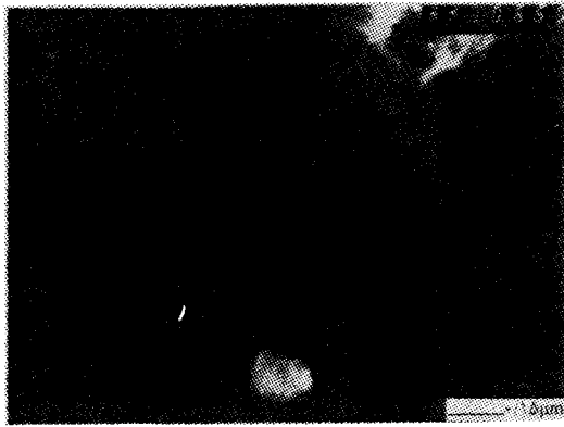
شکل ۱۹: ساختار میکروسکوپی از نقطه (۱۱۲) از الگوی پراش شکل ۱۸. میدان تاریک.
