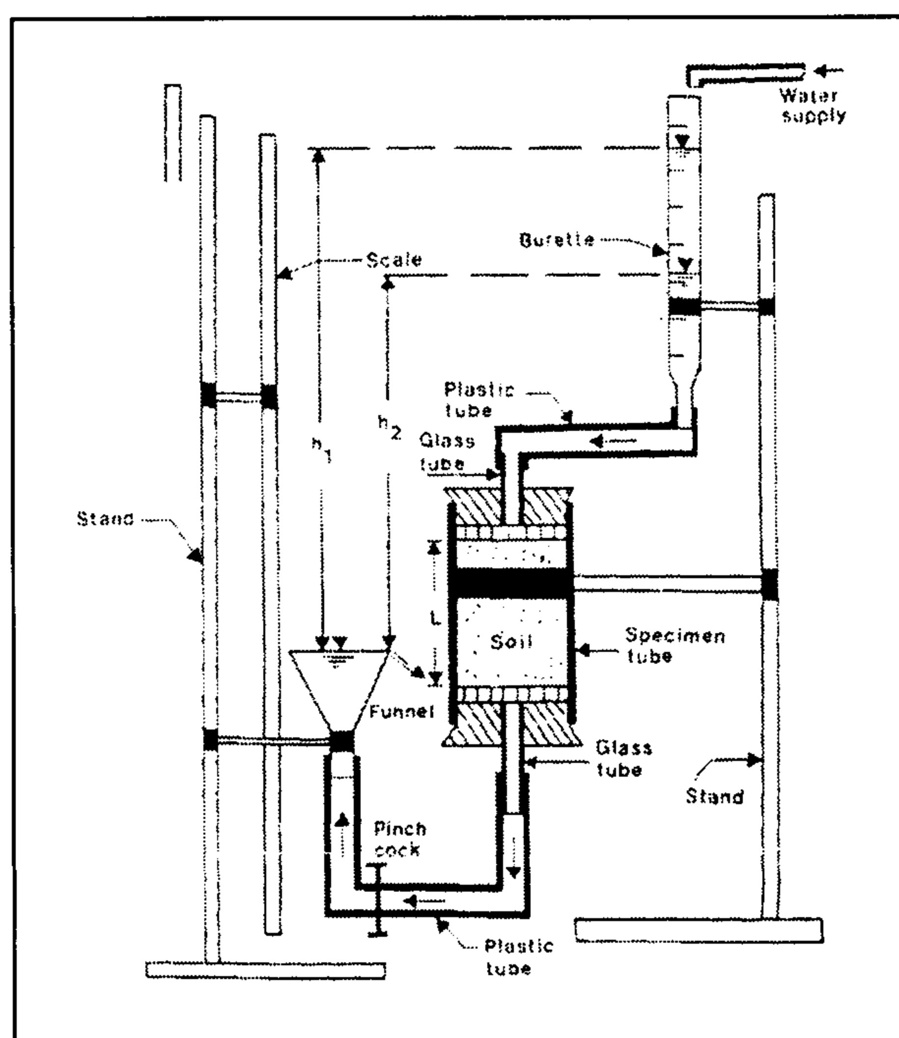
شکل شماره (۱): تصویر شماتیک از دستگاه آزمایش نفوذپذیری با هد متغیر (Das, 1990)
