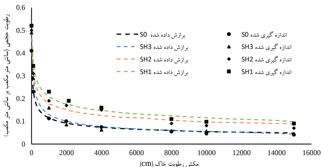
شکل ۴. منحنی مشخصه رطوبتی خاک شاهد و خاک اصلاح شده با هیدروچار در اندازه ذرات مختلف
