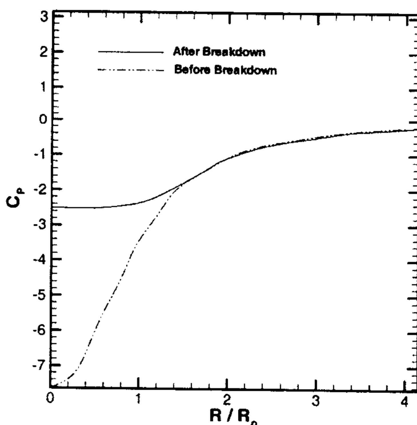
شکل ۷: تغییرات ضریب فشار استاتیک با شعاع هسته.
