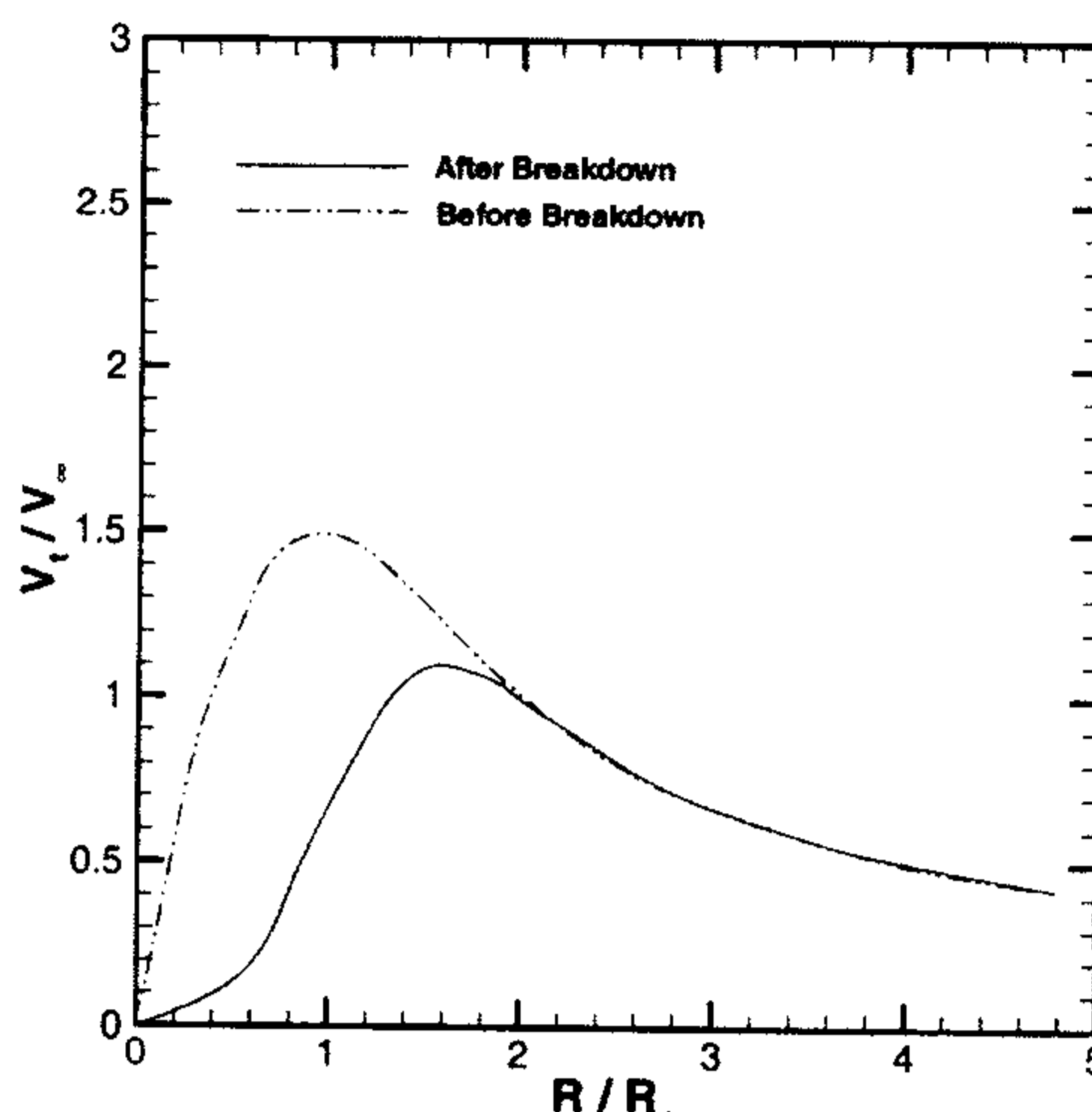
شکل ۵: تغییرات سرعت مماسی با شعاع هسته.
