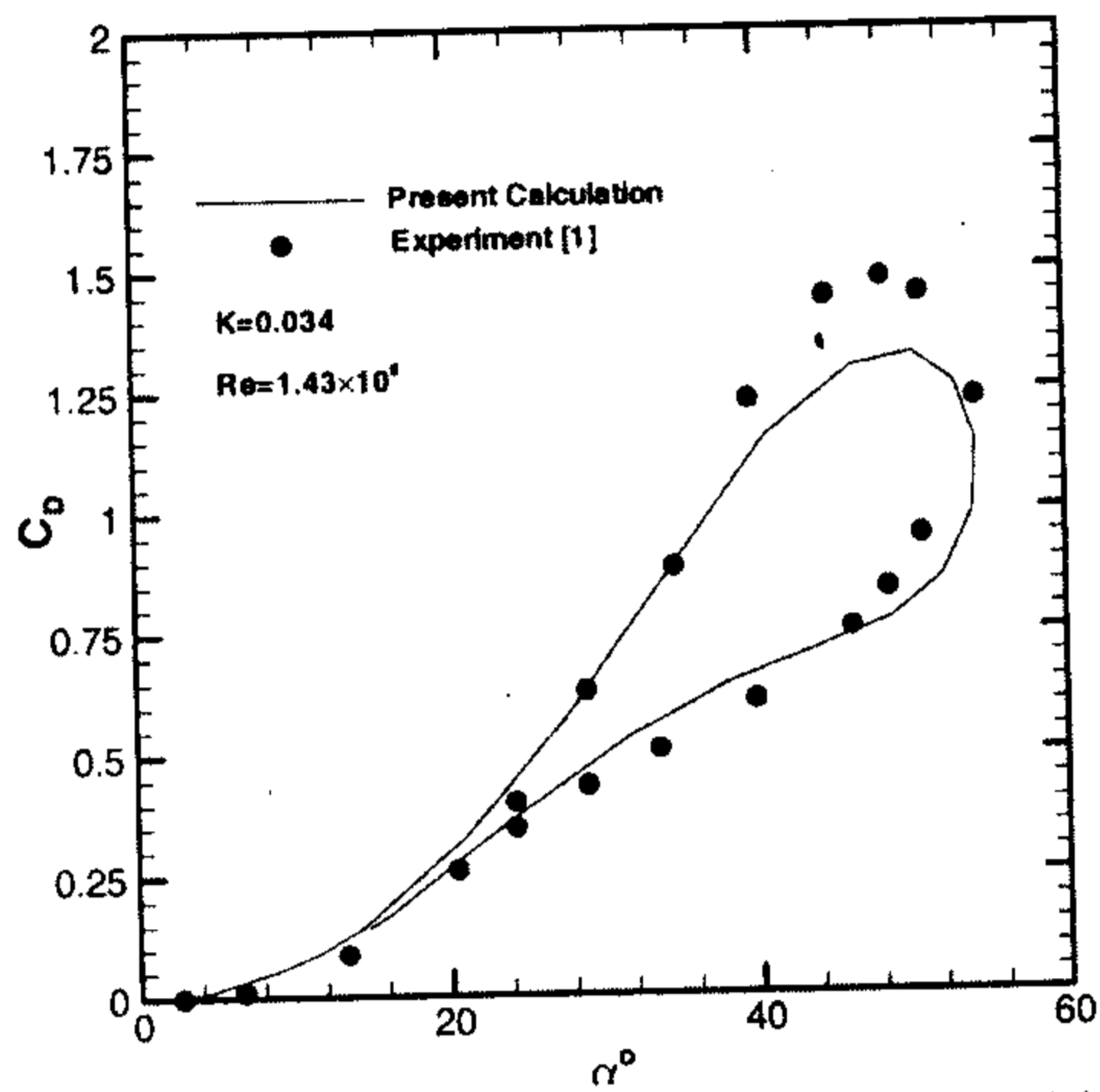
شکل ۱۲: تغییرات ضریب نیروی پسا با زاویه حمله.
