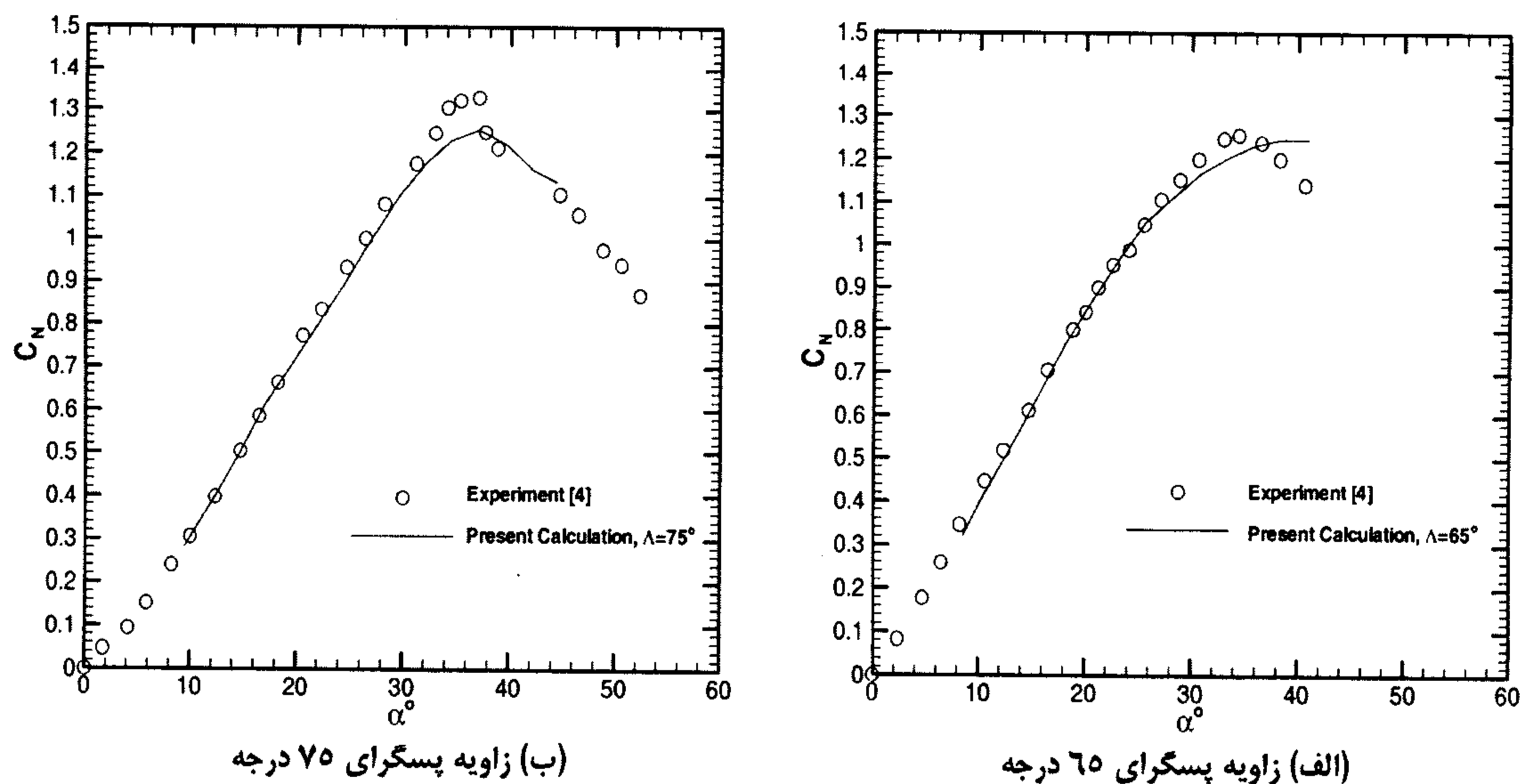
شکل ۱۰: تغییرات ضریب نیروی عمودی استاتیک با زاویه حمله.
