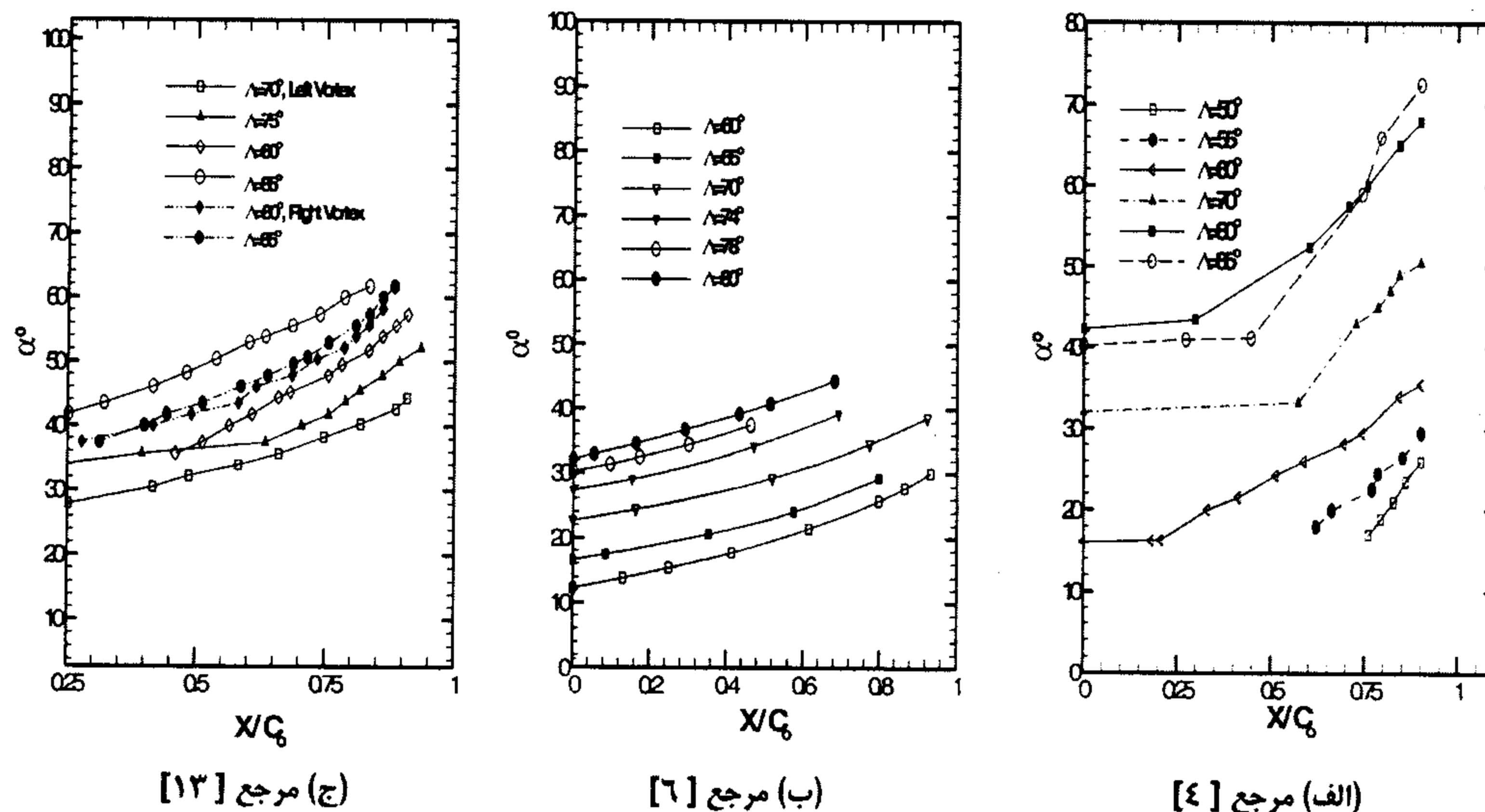
شکل ۹: تغییرات موقعیت نقطه انفجار با زاویه حمله.
