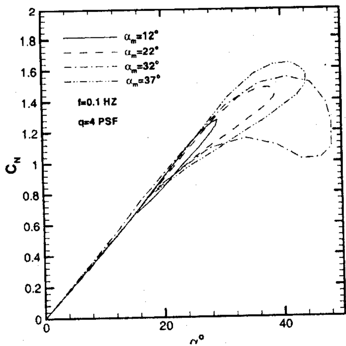
شکل ۱۶: اثر زاویه حمله متوسط روی تغییرات ضریب نیروی عمودی با زاویه حمله.
