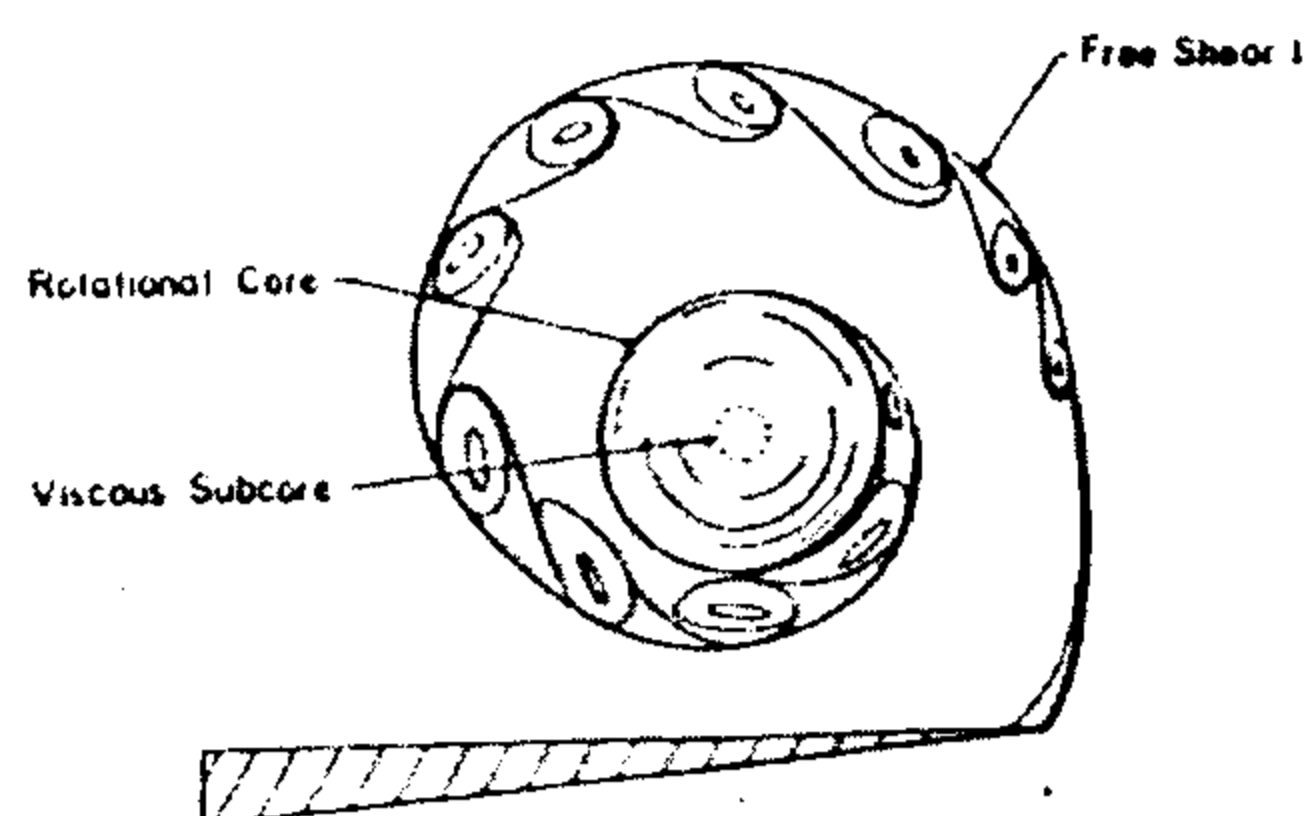
شکل ۲: نواحی مختلف درون گردابه [۱۳].
