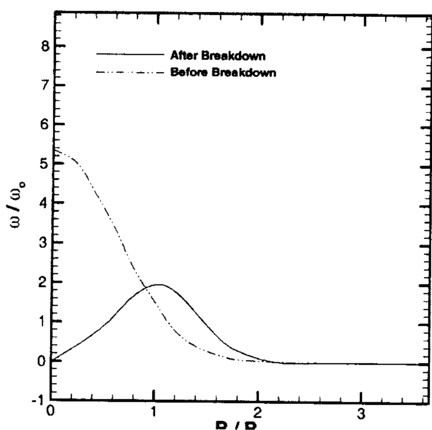
شکل ۶: تغییرات چرخش با شعاع هسته.
