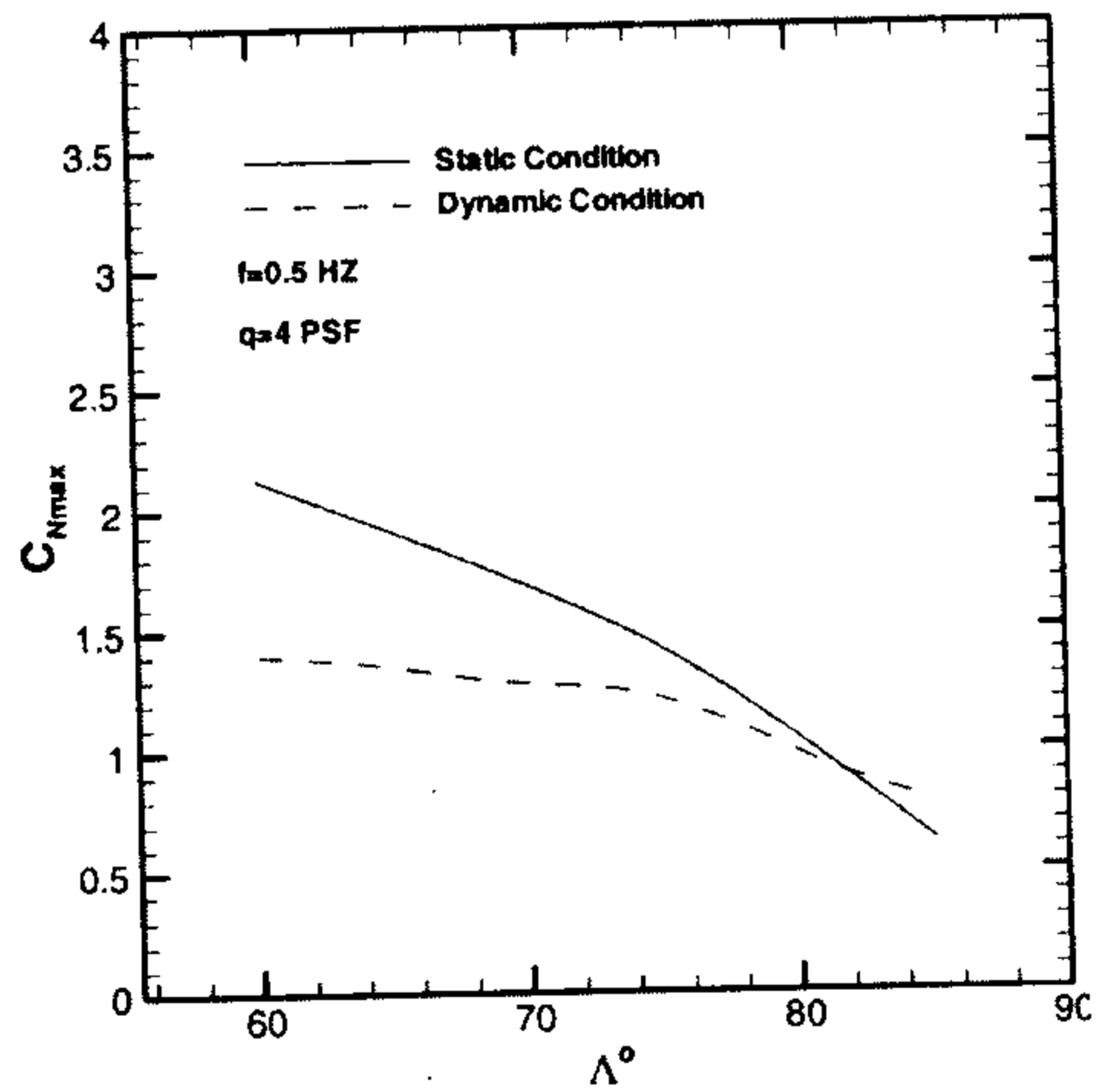
شکل ۱۳: تغییرات ضریب نیروی عمودی ماکزیمم.
