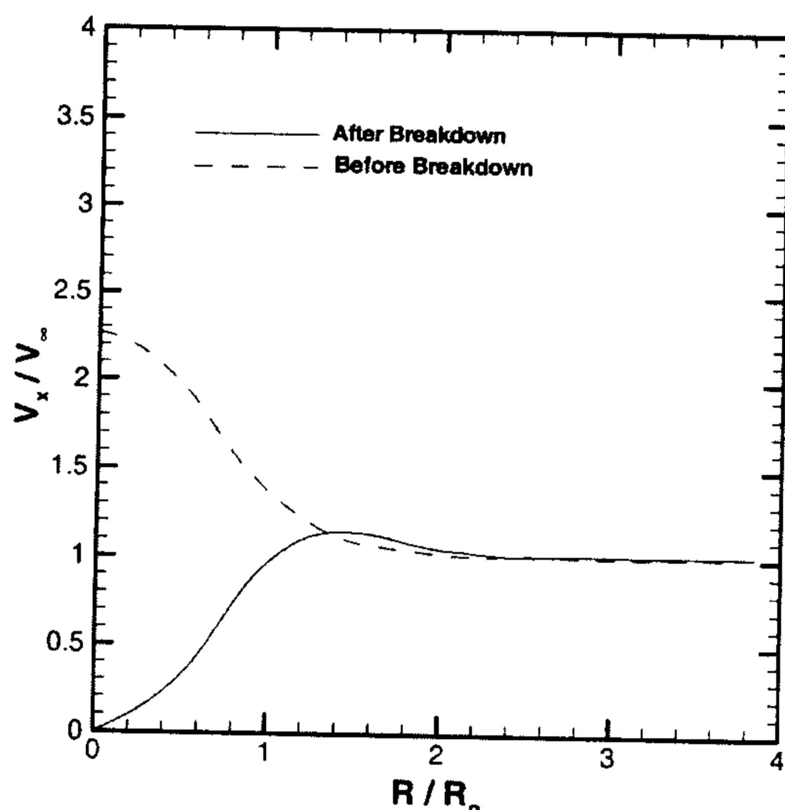
شکل ۴: تغییرات سرعت محوری با شعاع هسته.
