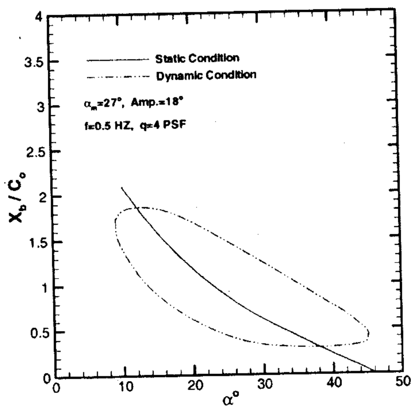
شکل ۱۴: تغییرات موقعیت نقطه انفجار با زاویه حمله.
