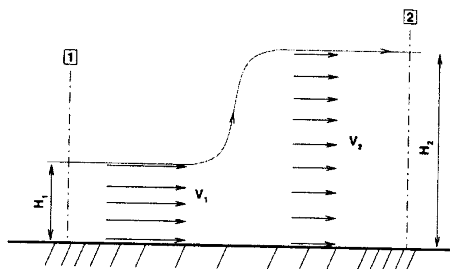
شکل ۳: مفهوم پرش هیدرولیکی [۱۵].
