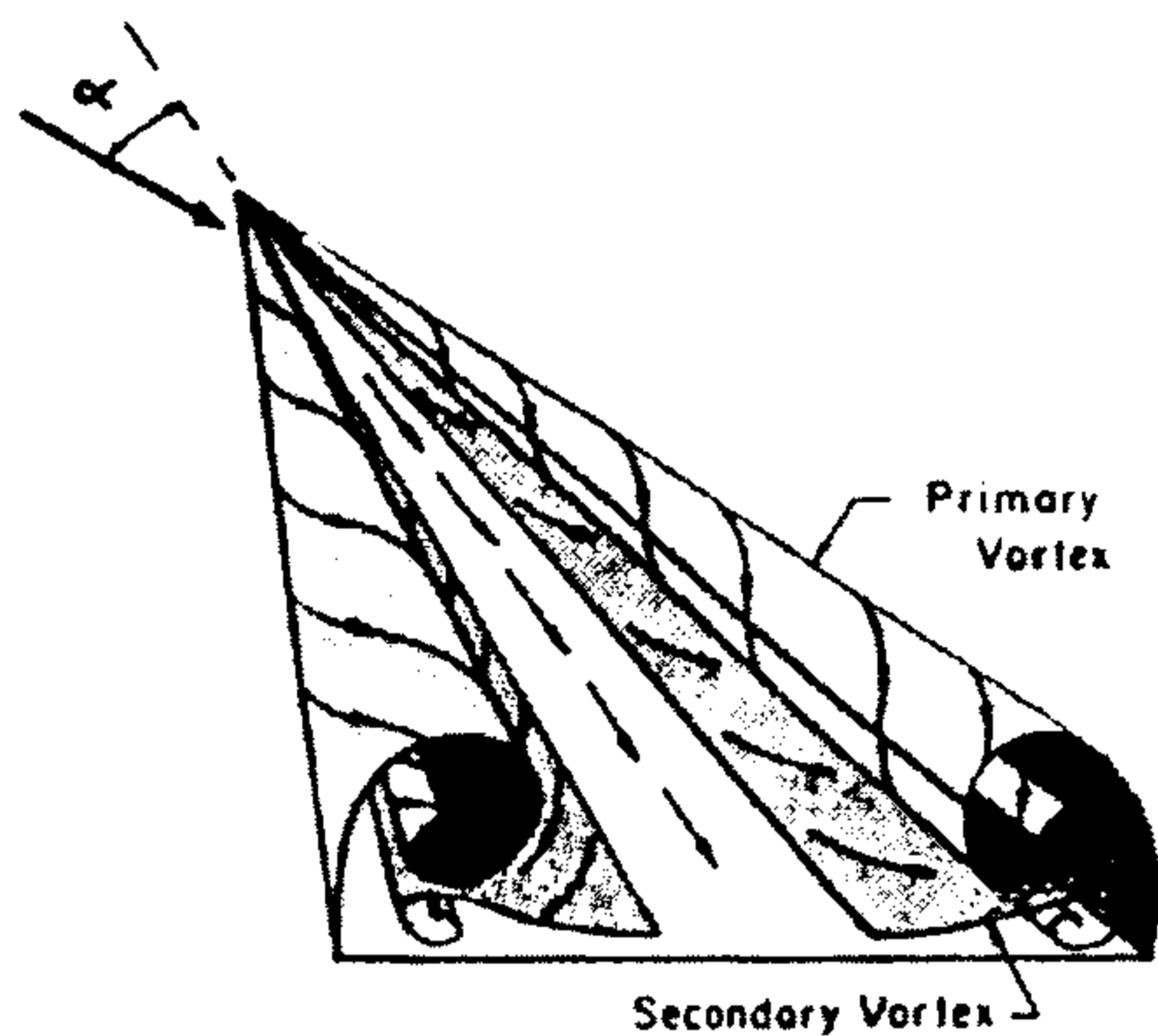
شکل ۱: گردابه‌های لبه حمله روی یک بال مثلثی [۱].
