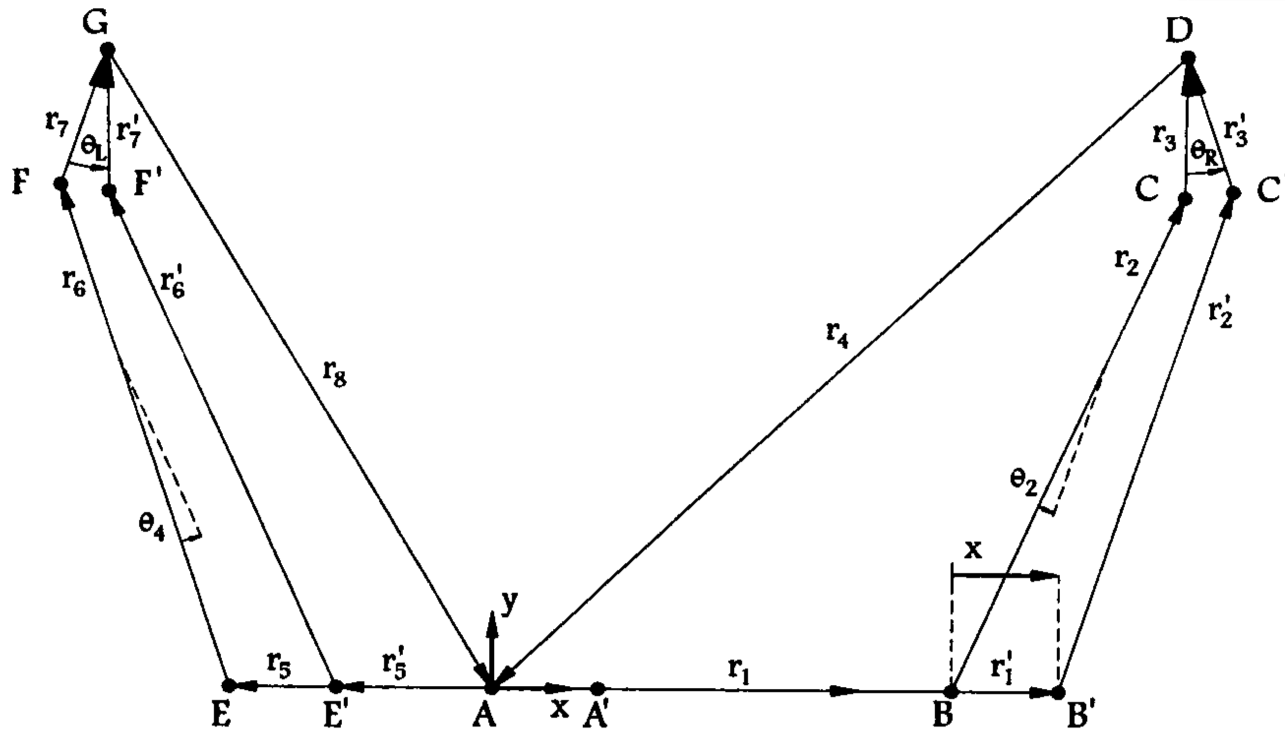
شکل ۳: مدل سینماتیکی فرمان.
