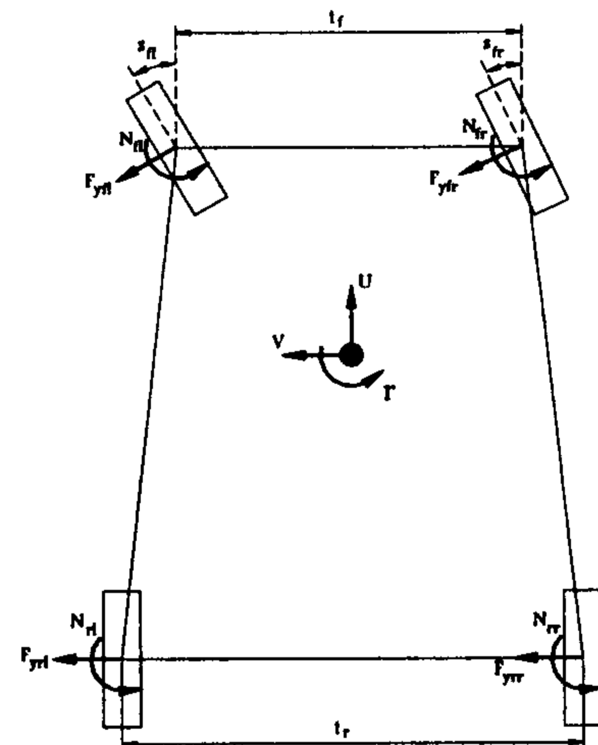
شکل ۱: مدل دینامیکی خودرو.
