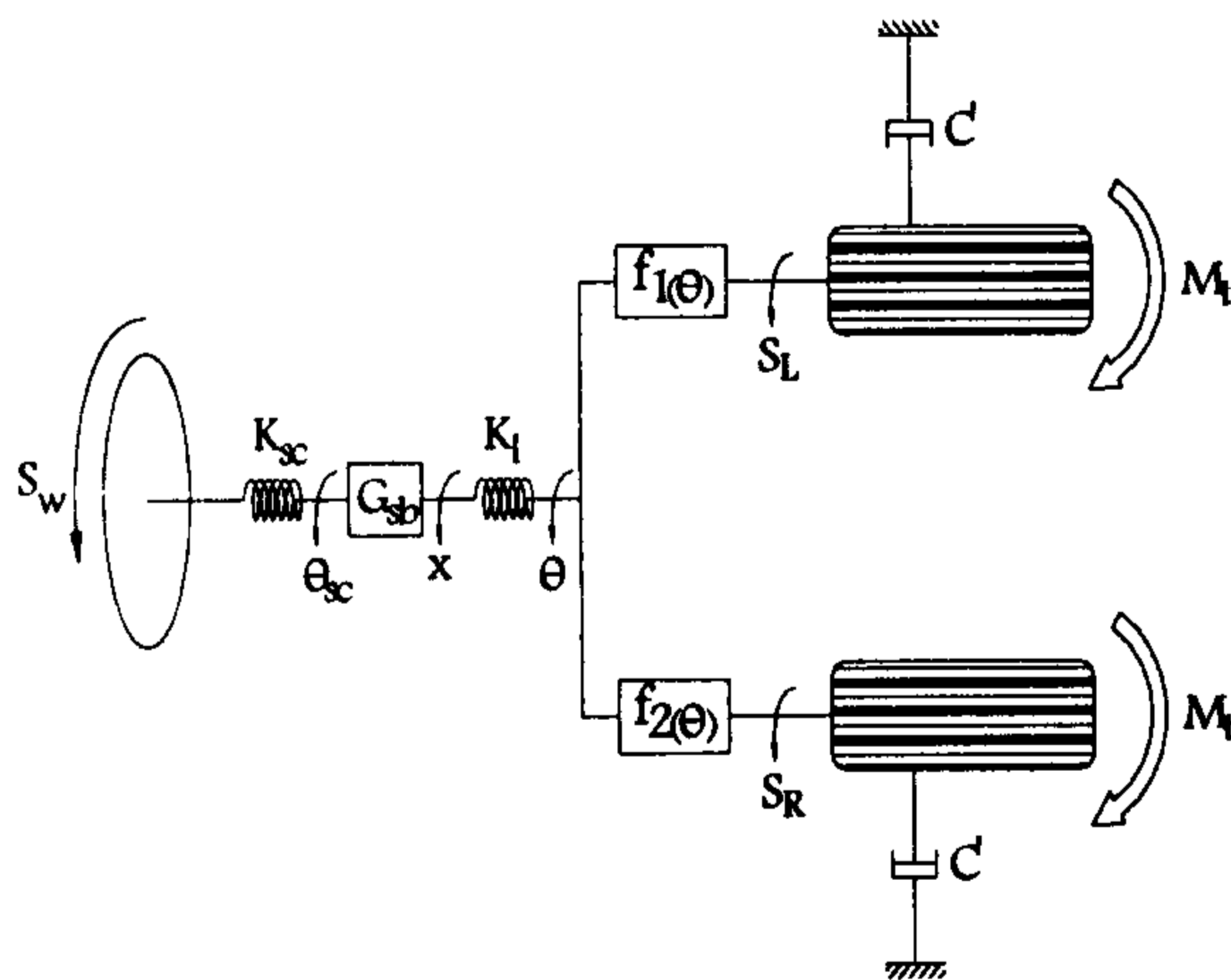
شکل ۲: مدل دینامیکی فرمان.
