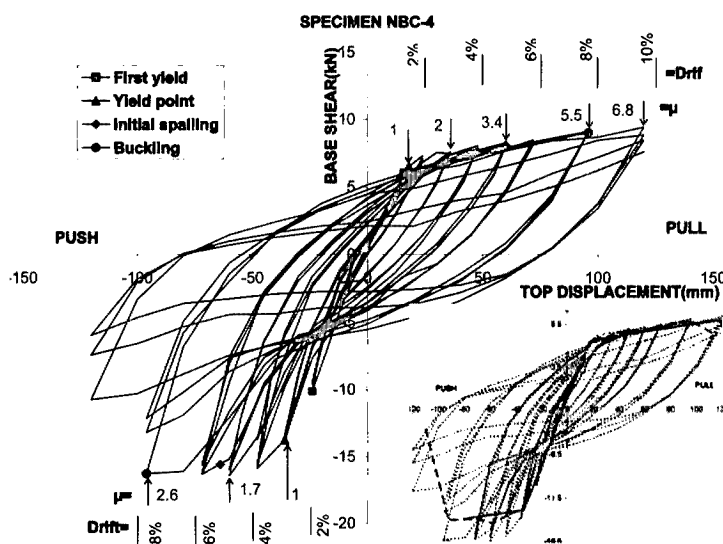
شکل ۵: نمودار دررفت-مقاومت جانبی برای نمونه نیمه مهندسی تیر طبقات زیرین، NBC-4.
