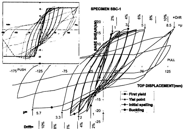
شکل ۹: نمودار مقاومت جانبی در برابر تغییر شکل برای نمونه 1 - SBC.
