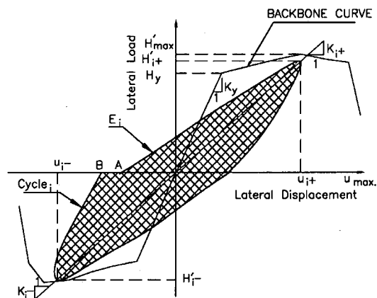
شکل ۱۴: منحنی نمایش استهلاک انرژی.
