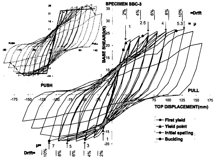
شکل ۷: نمودار مقاومت جانبی در برابر تغییر شکل برای نمونه 3 - SBC.
