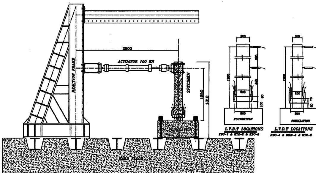
شکل ۲: نمایی از ابزار بندی آزمایش.
