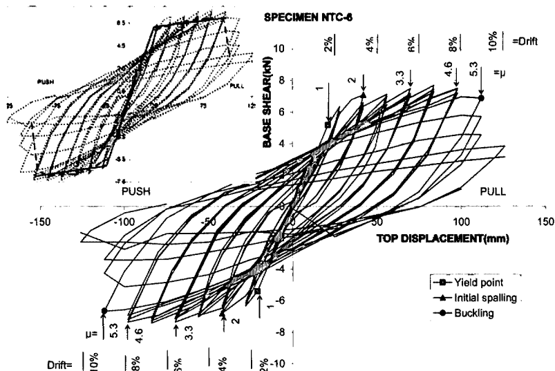
شکل ۴: نمودار تغییرشکل-مقاومت جانبی برای نمونه نیمه مهندسی تیر طبقات فوقانی، NTC-6.
