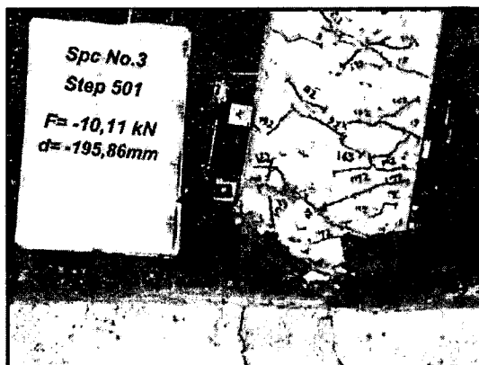
شکل ۱۰: نحوه تخریب در نمونه SBC-3 (الف) در جابه‌جایی جانبی ۶۴ میلی‌متر (ب) انتهای بارگذاری.
