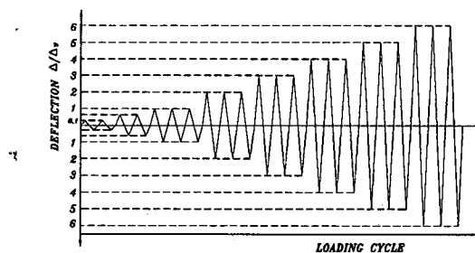
شکل ۳: رویه بارگذاری نمونه‌ها.
