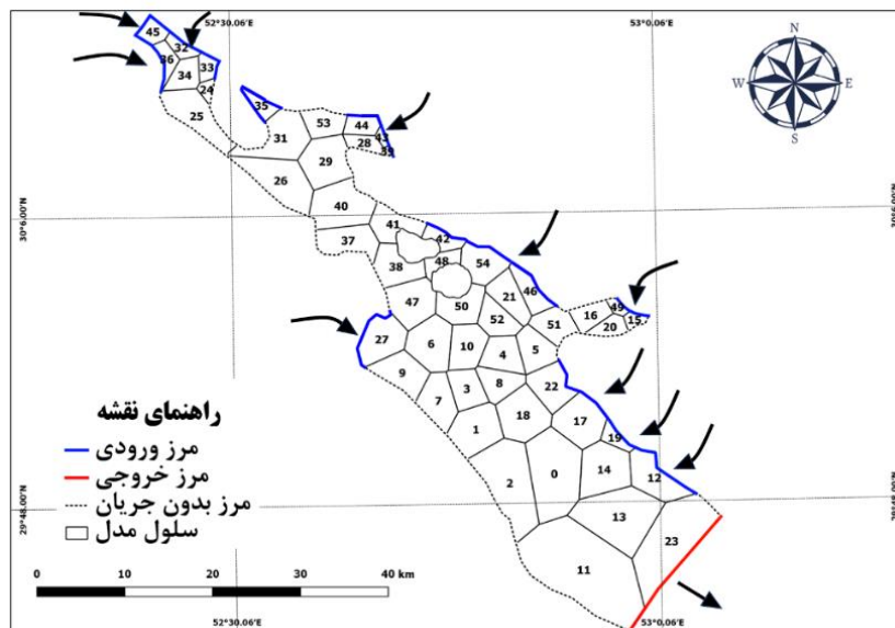
شکل ۵. مرزهای ورود و خروج جریان زیرزمینی
