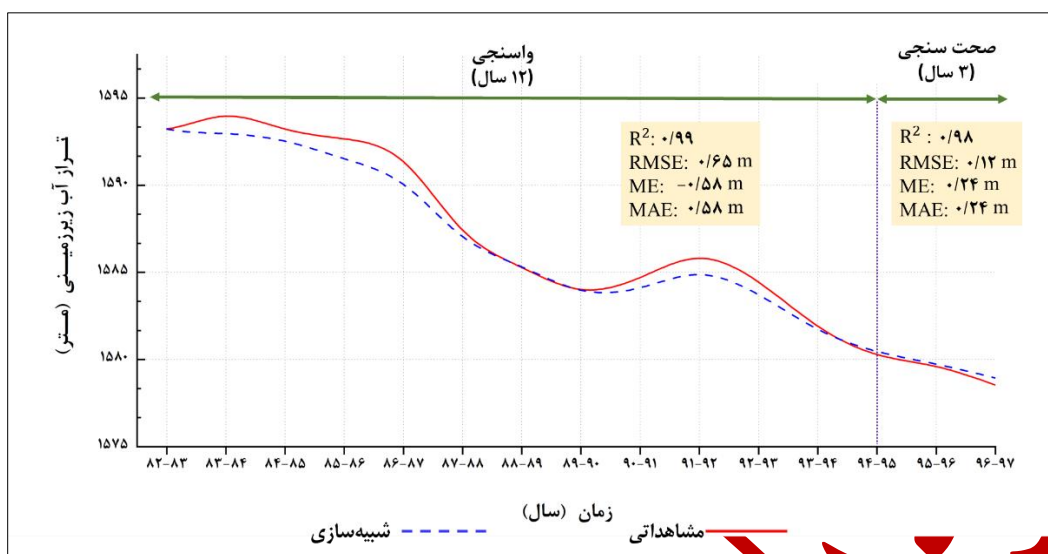
شکل ۱۲. مقایسه تراز محاسباتی و تراز مشاهداتی آب زیرزمینی در دوره واسنجی و صحت‌سنجی مدل
