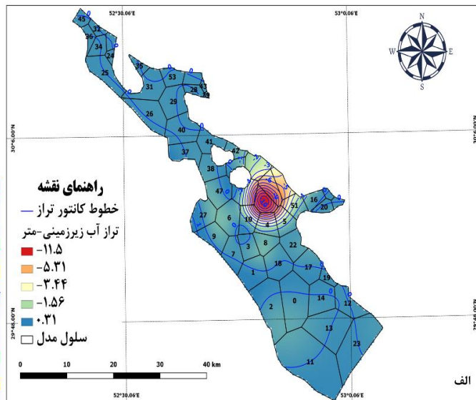
شکل ۲۰ الف: نقشه اختلاف هم تراز آب زیرزمینی نسبت به وضعیت پایه، ب: هیدروگراف سلول، ج: جدول بیلان آبخوان
