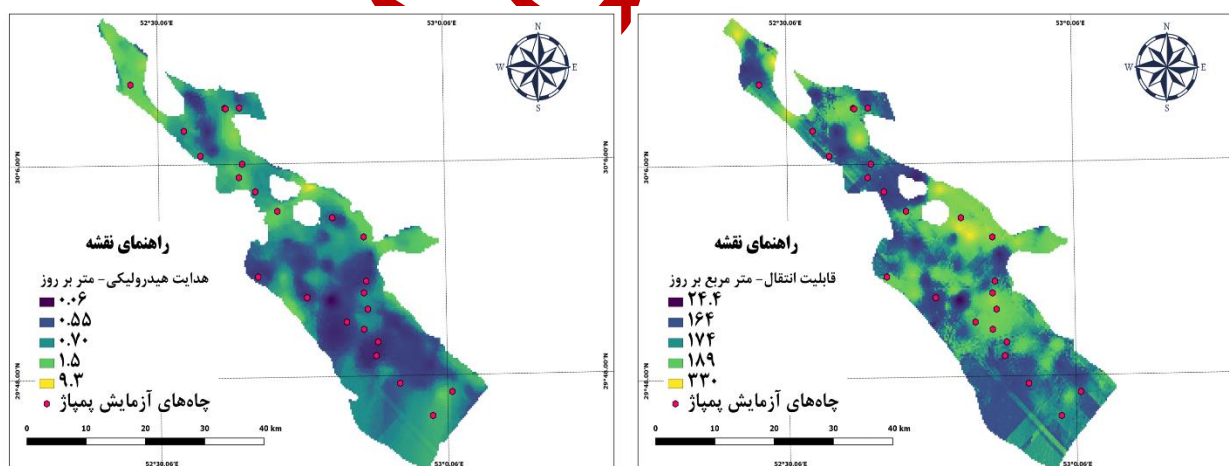
شکل ۱۳. الف: نقشه واسنجی شده قابلیت انتقال و ب: نقشه واسنجی شده هدایت هیدرولیکی
