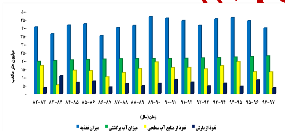
شکل ۱۵. مقادیر بدست آمده از پارامترهای واسنجی شده در طول دوره شبیه‌سازی
