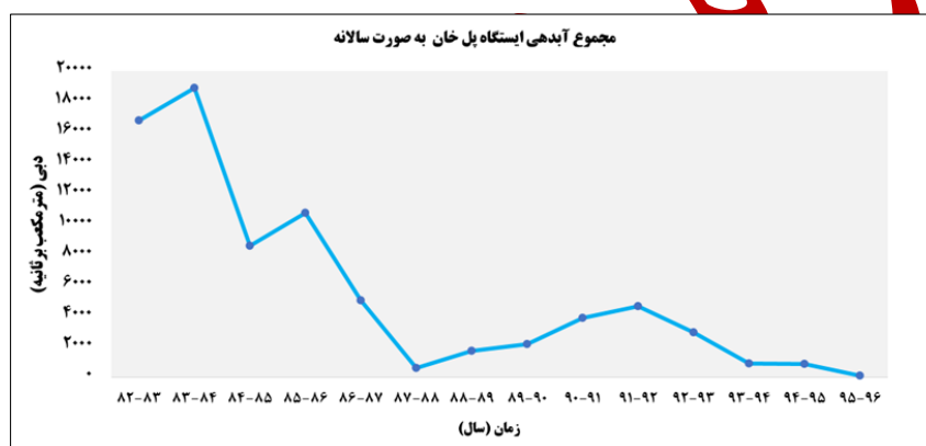
شکل ۵. میزان آبدهی ایستگاه پل خان
