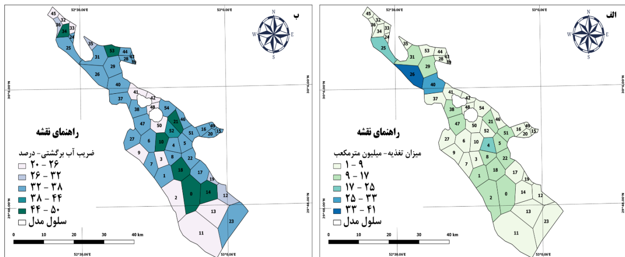
شکل ۱۴. الف: میزان تغذیه واسنجی شده و ب: میزان ضریب آب برگشتی واسنجی شده در سلول‌های محدوده
