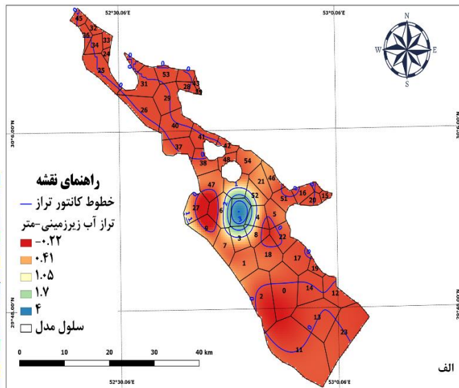
شکل ۱۸ الف: نقشه اختلاف هم تراز آب زیرزمینی نسبت به وضعیت پایه، ب: هیدروگراف سلول، ج: جدول بیلان آبخوان
