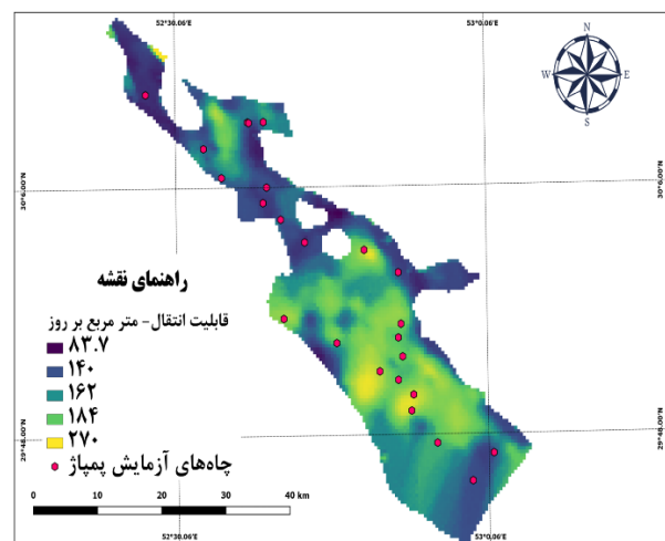
شکل ۷. الف: نقشه قابلیت انتقال و ب: نقشه هدایت هیدرولیکی
