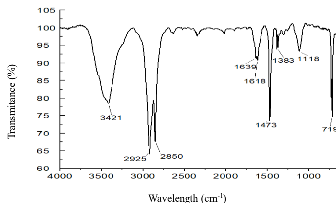
شکل ۱- طیف سنجی مادون قرمز پلی اتیلن سنگین
