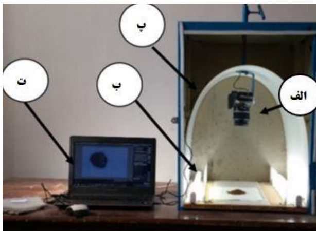
شکل ۲: نمایی از چیدمان تصویربرداری (الف) دوربین (ب) منبع نور فلورسنت (پ) صفحه قوسی (ت) رایانه
