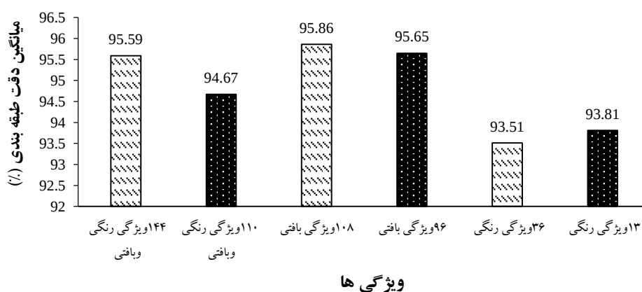
شکل ۸: مقایسه میانگین دقت طبقه بندی نمونه‌ها با استفاده از ویژگی‌های ترکیبی (بافتی-رنگی) با ویژگی‌های بافتی و رنگی به صورت مجزا
