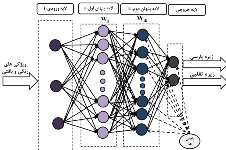
شکل ۶: ساختار شبکه عصبی MLP استفاده شده
