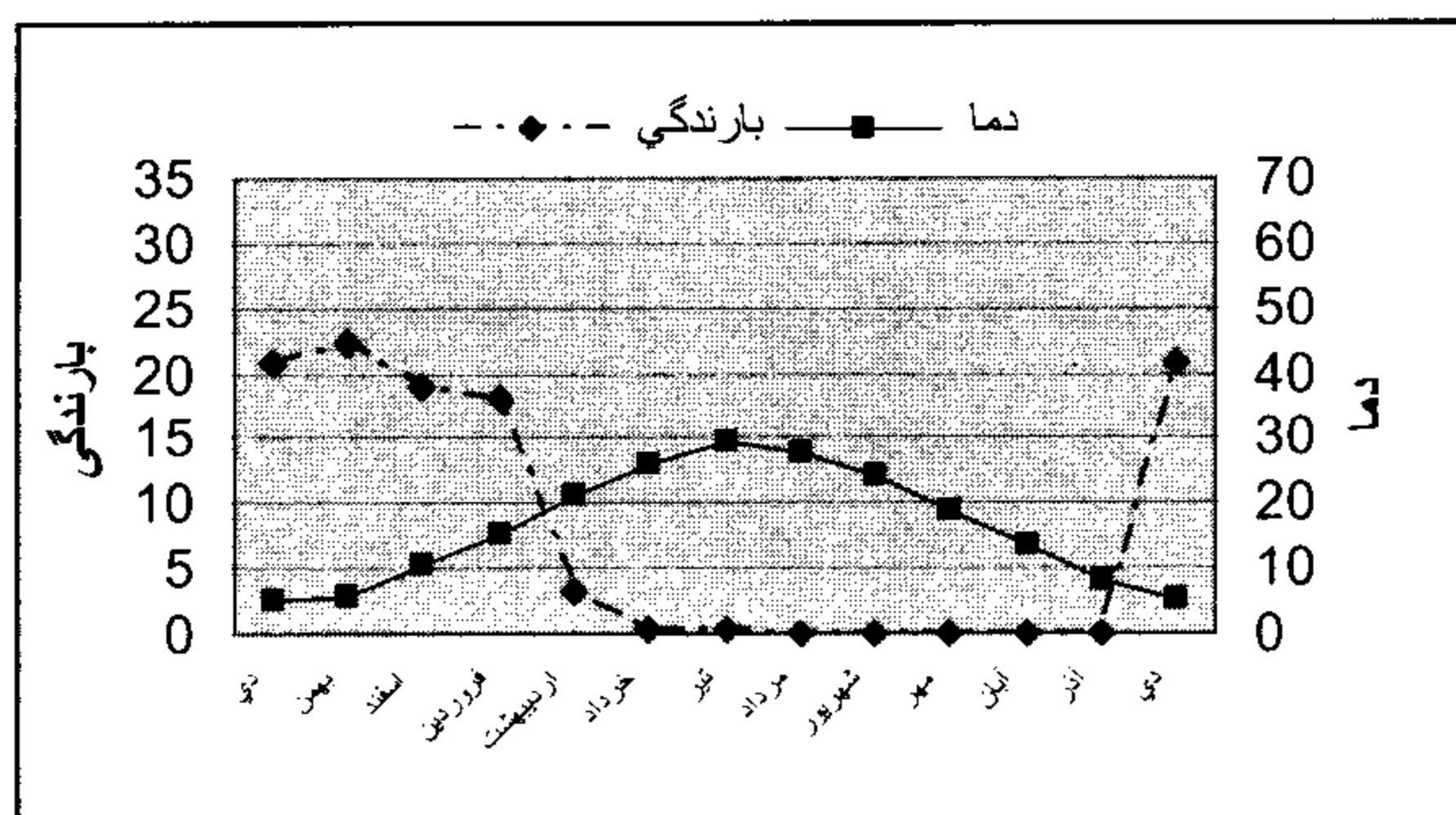
شکل شماره (۳): نمودار آمبروترمیک ایستگاه بافق
