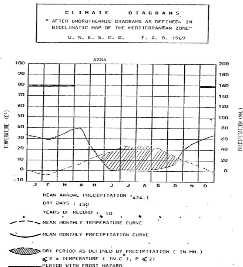
شکل ۲: منحنی آمبروترمیک منطقه
