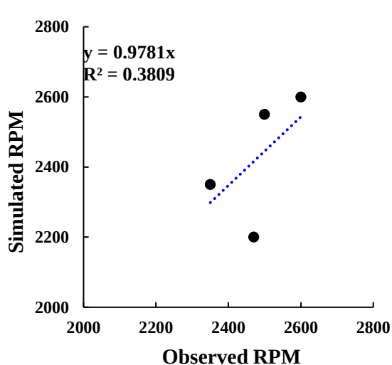
شکل ۱۴- تحلیل جامع عملکرد آبان‌ماه مدل MLP در پیش‌بینی دور پمپ چاه‌های آب شرب در مراحل آموزش و آزمون
