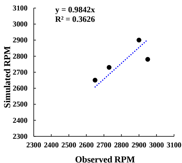
شکل ۱۱- تحلیل جامع عملکرد مردادماه مدل MLP در پیش‌بینی دور پمپ چاه‌های آب شرب در مراحل آموزش و آزمون
