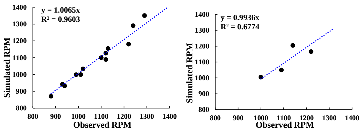
شکل ۱۸- تحلیل جامع عملکرد اسفندماه مدل MLP در پیش‌بینی دور پمپ چاه‌های آب شرب در مراحل آموزش و آزمون
