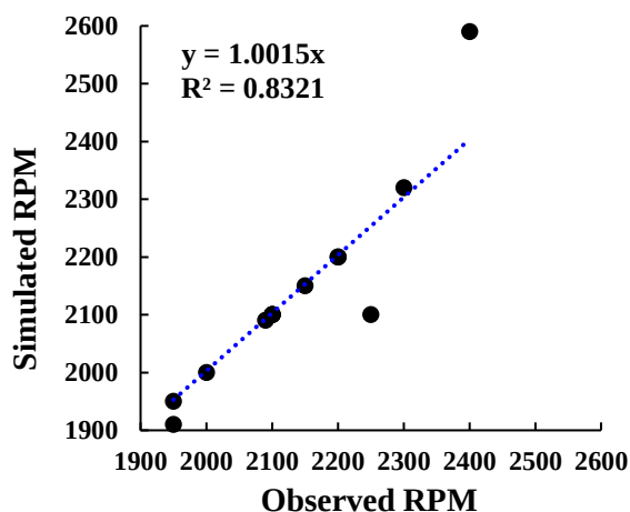
شکل ۱۰- تحلیل جامع عملکرد تیرماه مدل MLP در پیش‌بینی دور پمپ چاه‌های آب شرب در مراحل آموزش و آزمون
