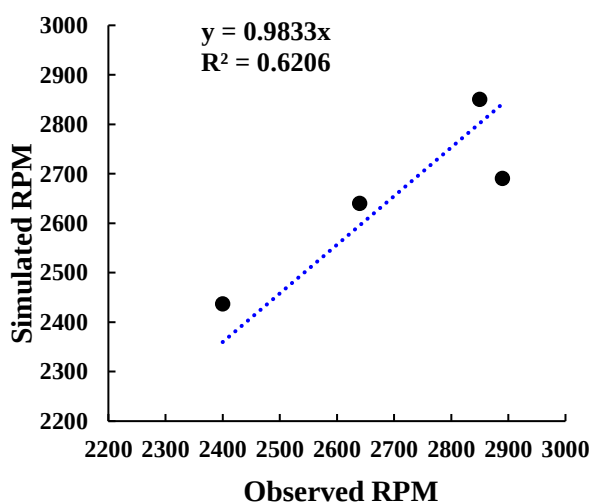
شکل ۱۲- تحلیل جامع عملکرد شهریورماه مدل MLP در پیش‌بینی دور پمپ چاه‌های آب شرب در مراحل آموزش و آزمون
