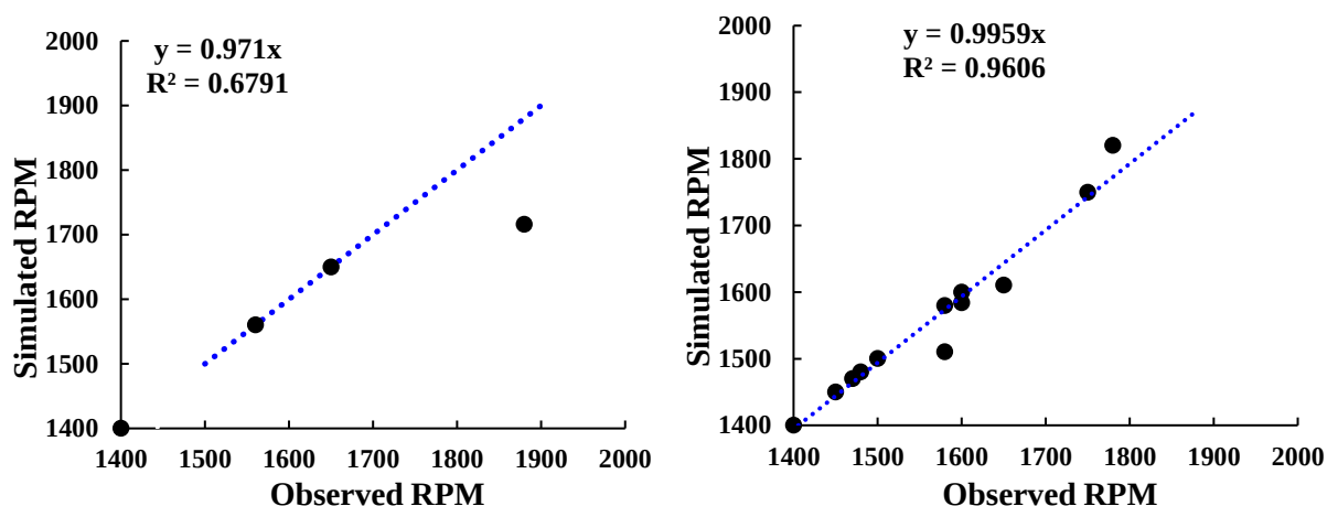
شکل ۱۶- تحلیل جامع عملکرد دی ماه مدل MLP در پیش‌بینی دور پمپ چاه‌های آب شرب در مراحل آموزش و آزمون
