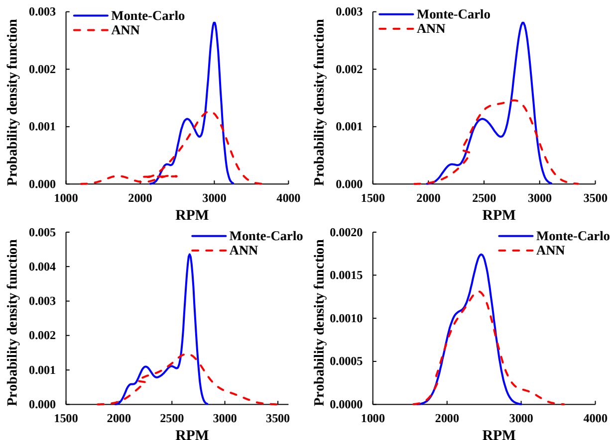
شکل ۲۰- مقایسه توزیع های احتمال RPM پیش بینی شده توسط شبکه عصبی و مونت کارلو برای ۴ ماه دوم سال
