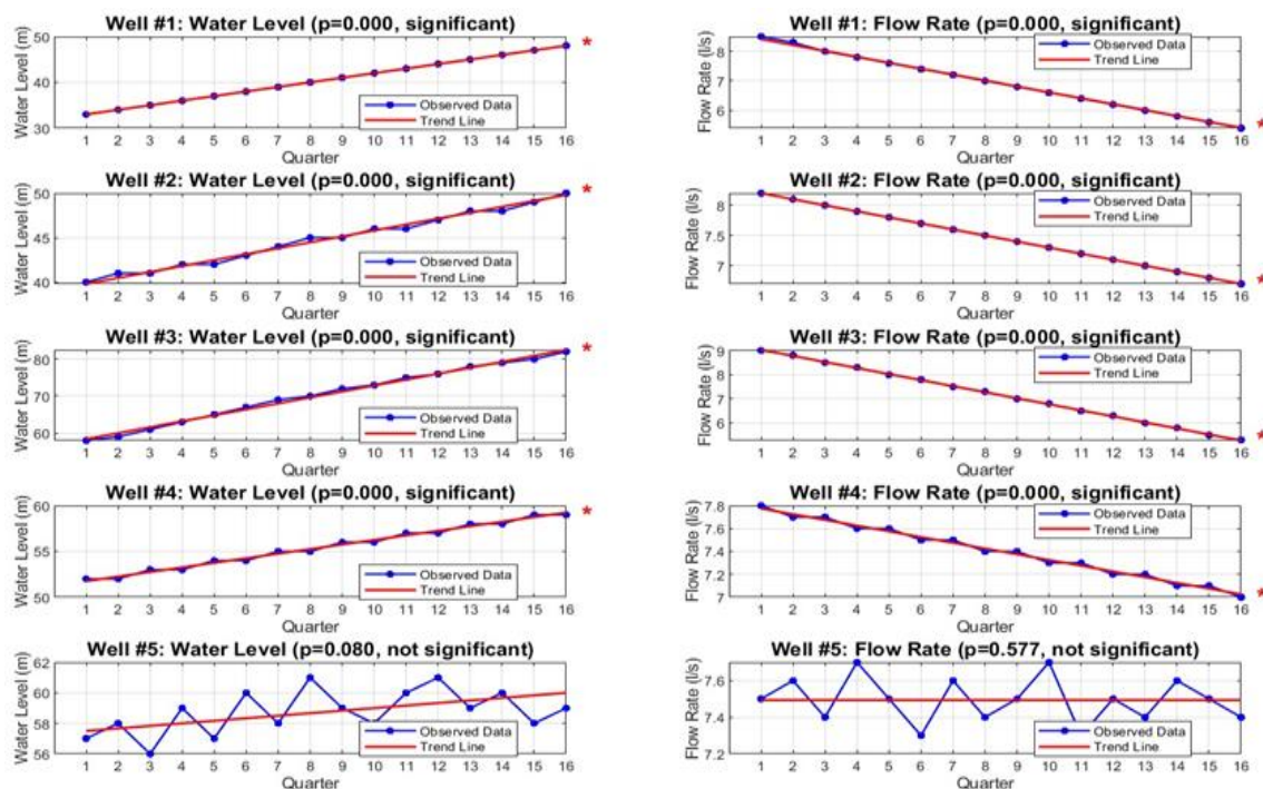
شکل ۶- نمایش سری‌های زمانی و خطوط روند برای پنج چاه مطالعاتی
