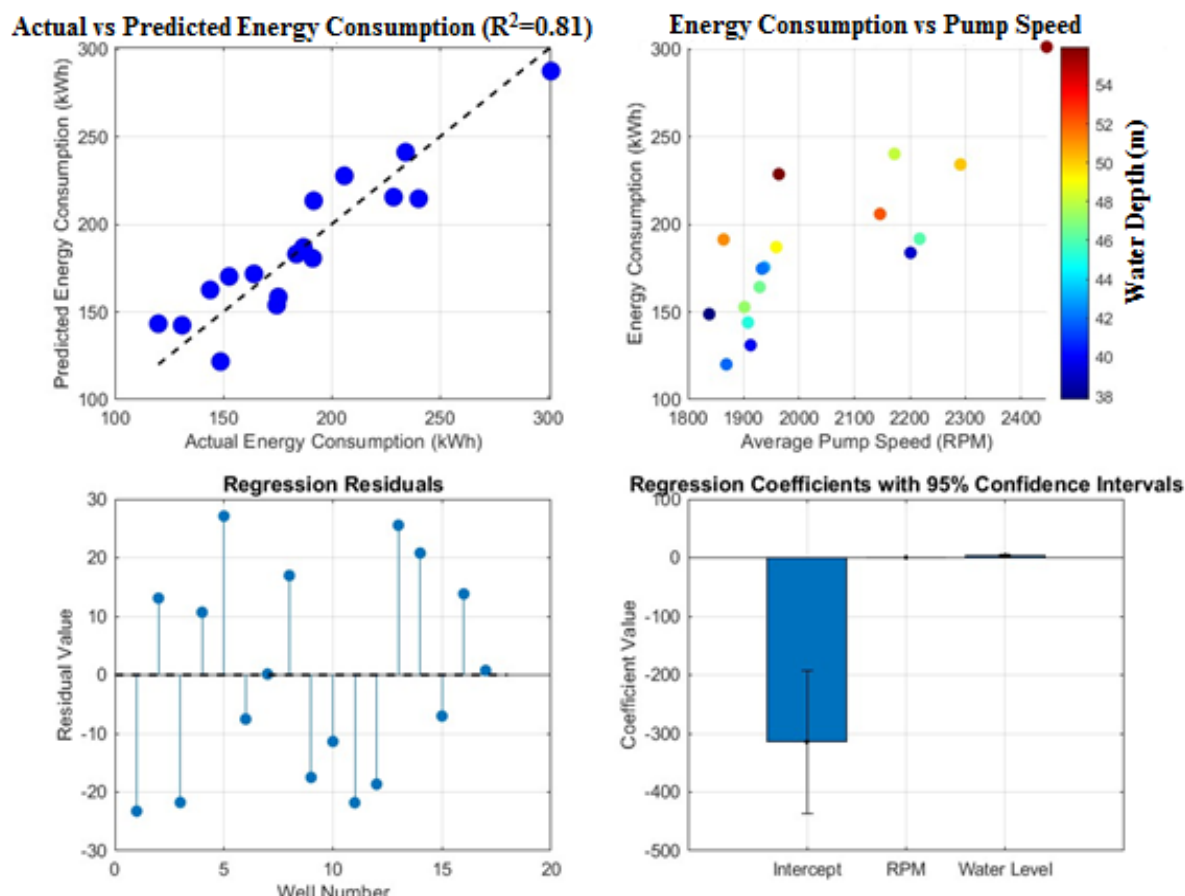
شکل ۵- آزمون رگرسیون خطی برای تعیین تأثیر دور پمپ و سطح آب بر مصرف انرژی
