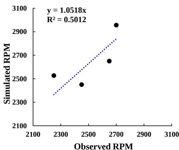
شکل ۱۳- تحلیل جامع عملکرد مهرماه مدل MLP در پیش‌بینی دور پمپ چاه‌های آب شرب در مراحل آموزش و آزمون
