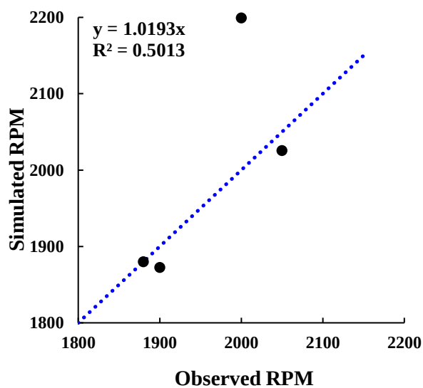
شکل ۱۵- تحلیل جامع عملکرد آذرماه مدل MLP در پیش‌بینی دور پمپ چاه‌های آب شرب در مراحل آموزش و آزمون
