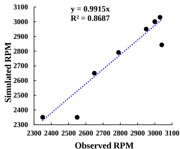
شکل ۱۱- تحلیل جامع عملکرد مردادماه مدل MLP در پیش‌بینی دور پمپ چاه‌های آب شرب در مراحل آموزش و آزمون
