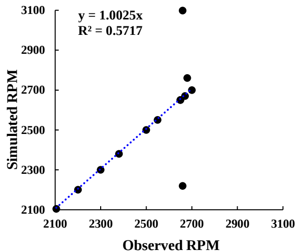
شکل ۱۳- تحلیل جامع عملکرد مهرماه مدل MLP در پیش‌بینی دور پمپ چاه‌های آب شرب در مراحل آموزش و آزمون
