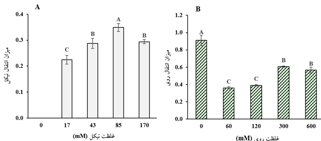
شکل ۴- اثر غلظت‌های مختلف نیکل و روی بر میزان انتقال آن‌ها در گیاه ریحان ( Ocimum basilicum ). هر عدد میانگین سه تکرار \pm انحراف از معیار که در شکل نشان داده شده است. حروف غیرمشابه، بیان‌گر اختلاف معنی‌دار بین داده‌ها براساس آزمون دانکن ( P < 0.05 ) است.
