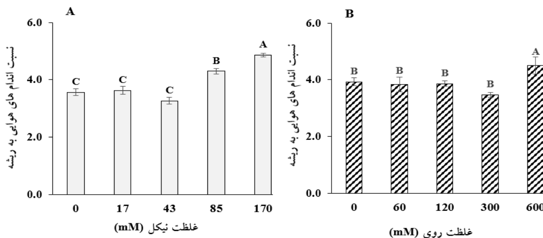
شکل ۲- اثر تنش نیکل و روی بر نسبت اندام‌های هوایی به ریشه (A, B) گیاه ریحان ( Ocimum basilicum ). هر عدد میانگین سه تکرار، \pm انحراف از معیار است. حروف غیرمشابه، بیان‌گر اختلاف معنی‌دار بین داده‌ها براساس آزمون دانکن ( P < 0.05 ) است.
