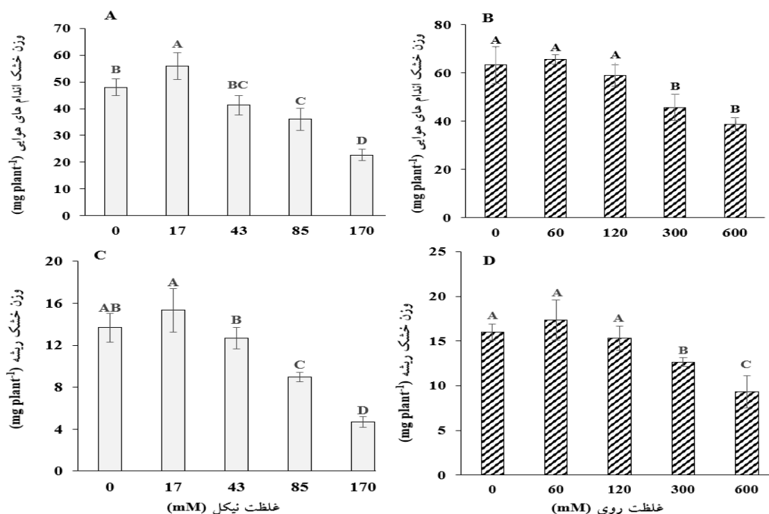
شکل ۱- اثر تنش نیکل و روی بر وزن خشک اندام های هوایی (A, B) و وزن خشک ریشه (C, D) ریحان ( Ocimum basilicum ). هر عدد میانگین سه تکرار، \pm انحراف از معیار است. حروف غیر مشابه، بیان گر اختلاف معنی دار بین داده ها براساس آزمون دانکن ( P < 0.05 ) است. پاسخ وزن خشک ریشه به غلظت های مختلف نیکل در شکل C-۱، نشان داد که وزن خشک ریشه گیاه ریحان مشابه با اندام های
