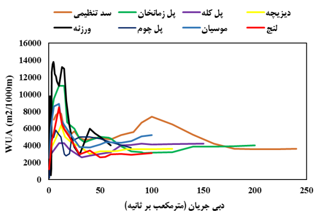
شکل ۷. نمودار دبی - فیزیکی زیستگاه در ایستگاه‌های مطالعاتی رودخانه زاینده‌رود
